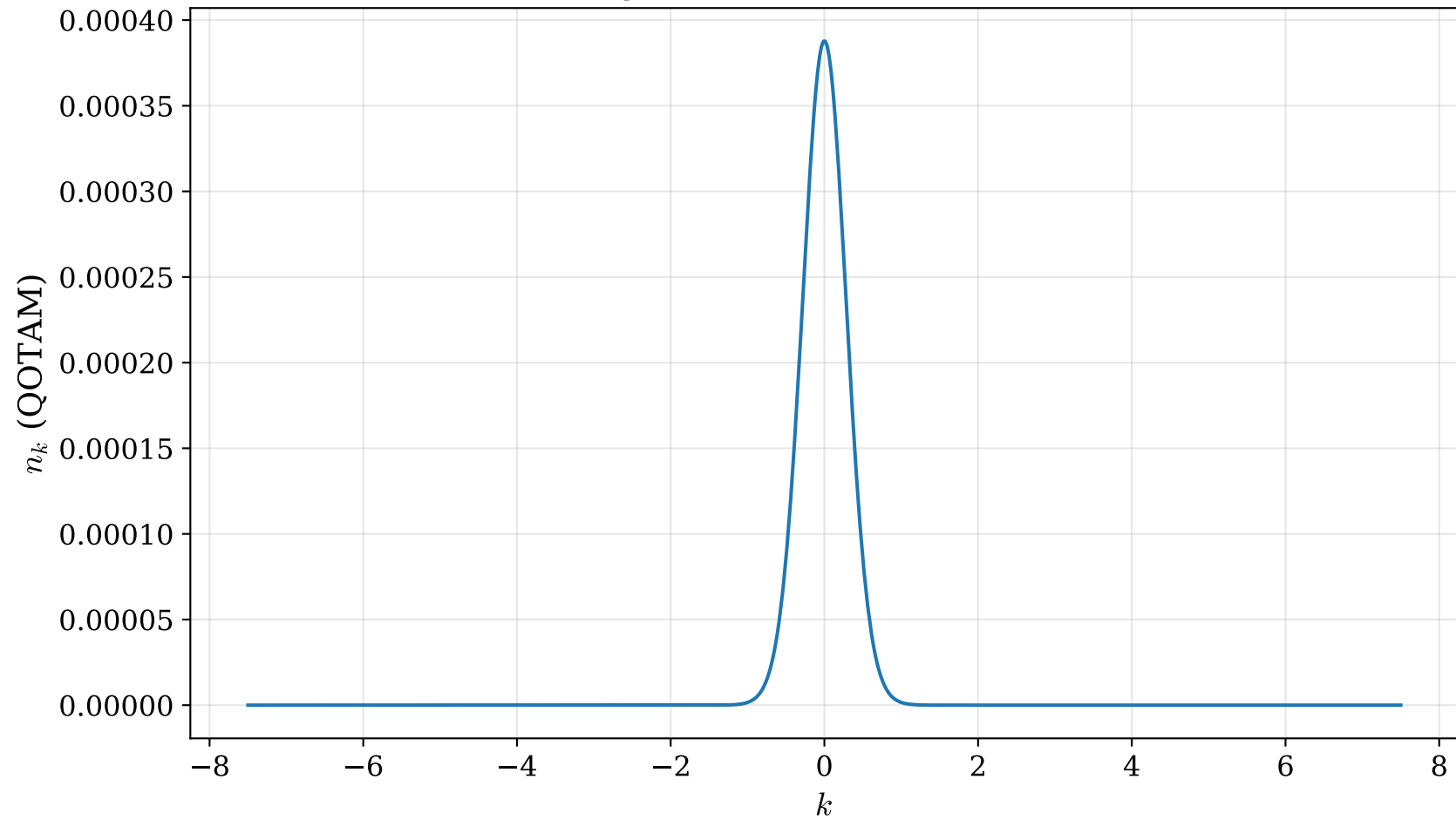
QOTAM Schwinger/Sauter spectrum ( E_0=0.300 , \tau=2.5 )
