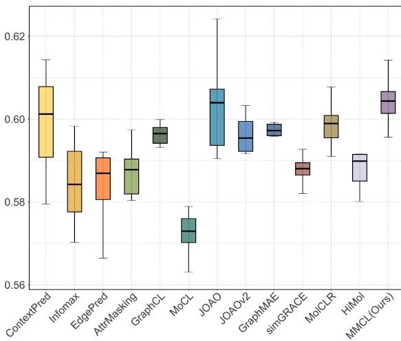
(d) SIDER
