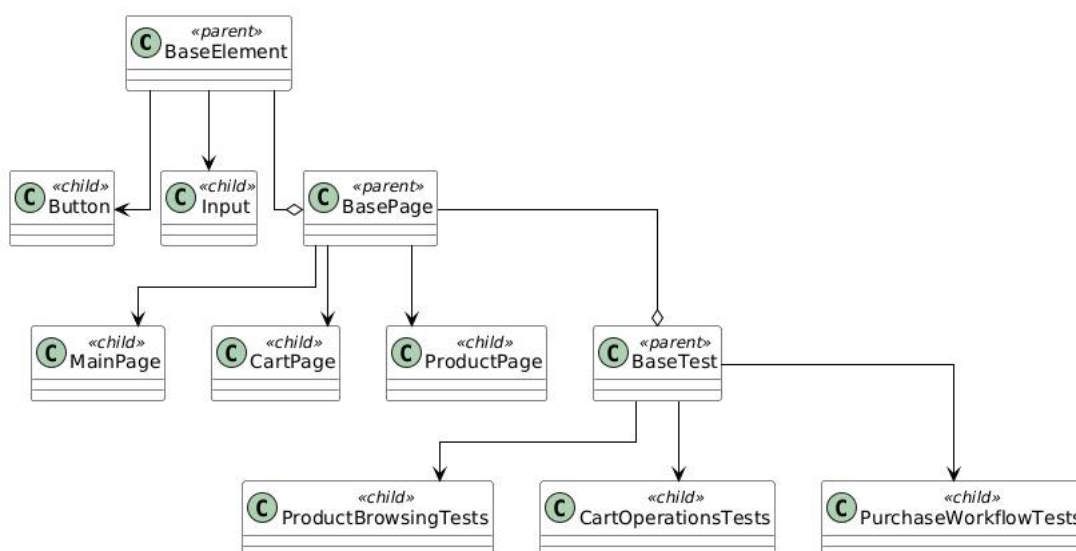
Рисунок 16 - UML-диаграмма
