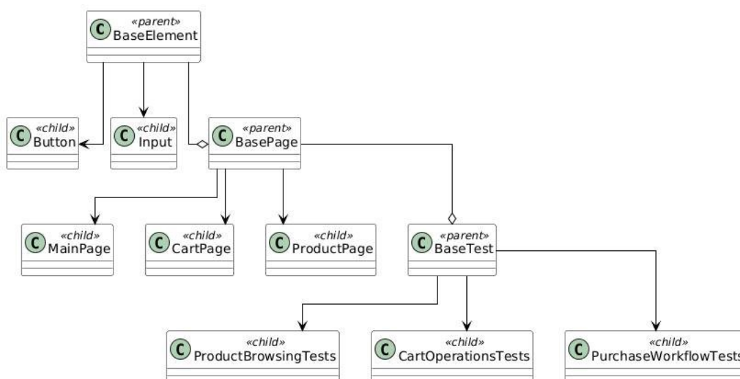
Рисунок 20 - UML-диаграмма
