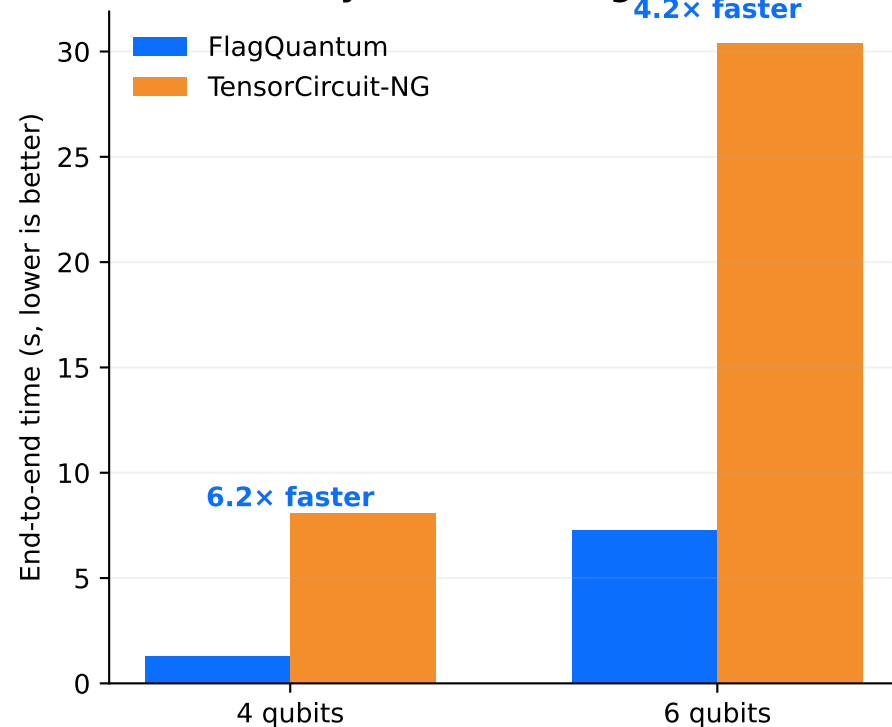
a Dynamic ansatz growth
