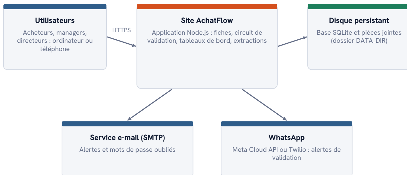
Schéma 1. Les pièces du système. Le site s'installe sur un hébergeur, avec un disque persistant qui conserve la base et les pièces jointes.
