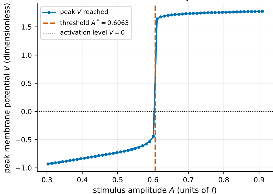
(d) Excitation threshold by bisection
