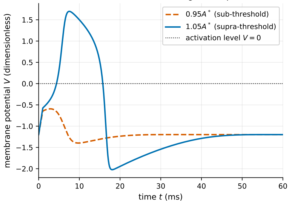
(d) Excitation threshold by bisection
