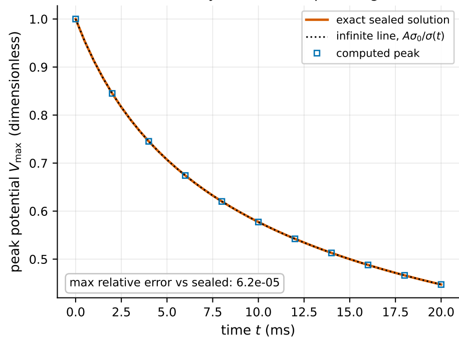
(d) Peak decay follows the spreading law
