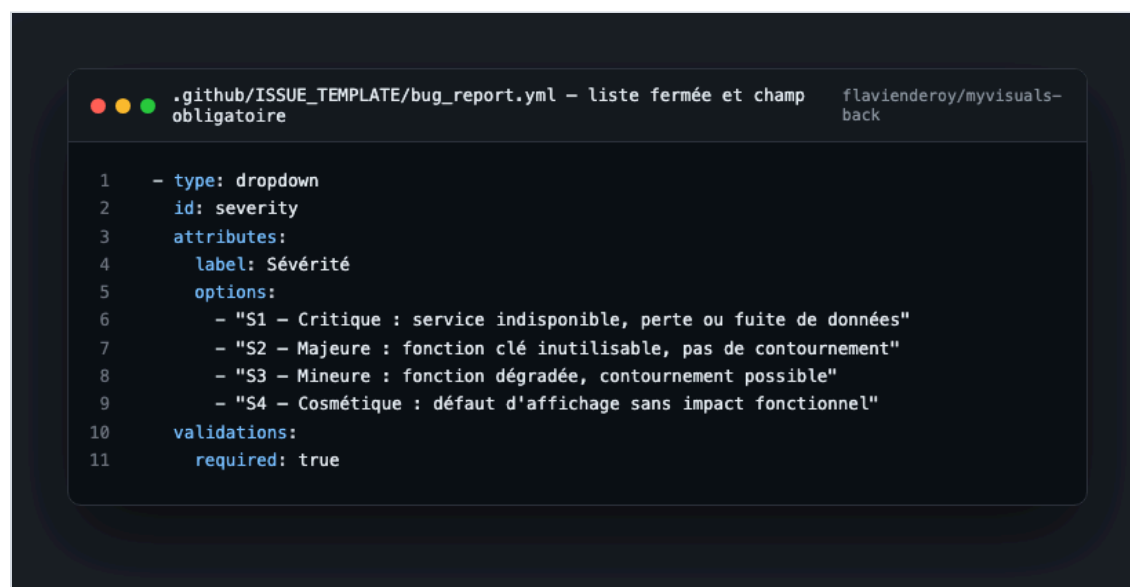
Figure 10 — Configuration du formulaire [ANO] : liste fermée et champ required: true . La sévérité — comme l'environnement, le composant et le canal de détection, construits à l'identique — ne peut pas être saisie librement : c'est ce qui rend les indicateurs de pilotage du § 2.3 calculables. Le formulaire une fois rempli figure ci-après.
