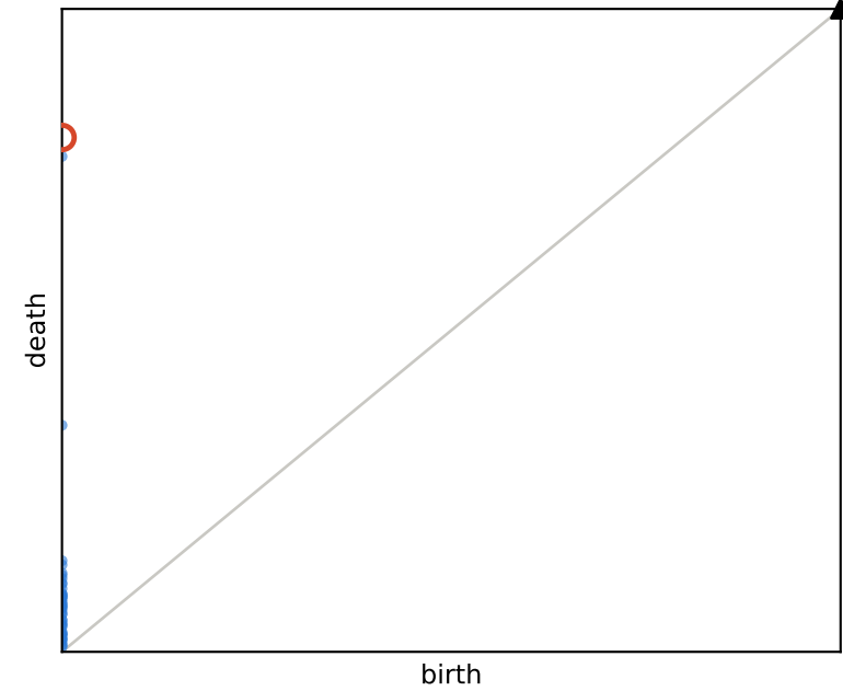
DTM 5 H_0
