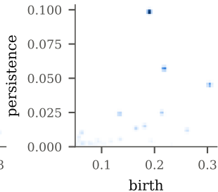
(f) PI H_1 , 64^2 , \sigma=0.5 px
