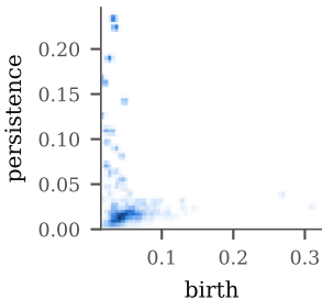
(e) PI H_0 , 64^2 , \sigma=0.5 px
