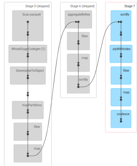
Figura 5. DAG di Spark per la Query 2: i tre job mostrano rispettivamente il filtraggio/aggregazione, il calcolo delle medie e l'ordinamento per il ranking top-10.
