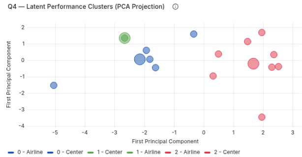
Figura 29. Risultati Query 4: Distribuzione geometrica dei cluster estratti tramite PCA.
