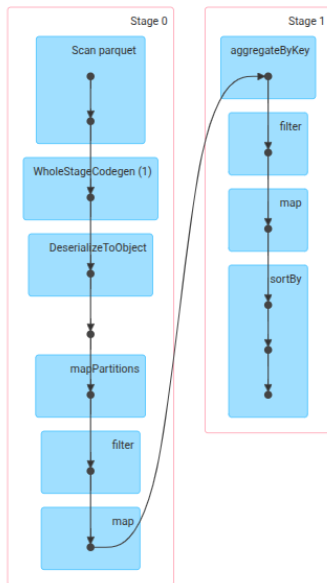
Figura 5. DAG di Spark per la Query 2: i tre job mostrano rispettivamente il filtraggio/aggregazione, il calcolo delle medie e l'ordinamento per il ranking top-10.
