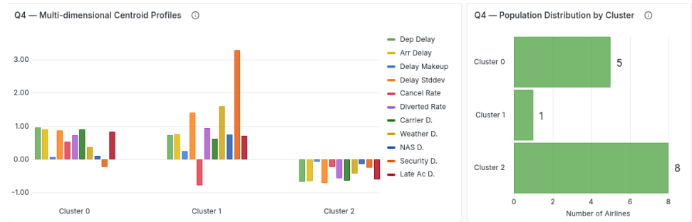
Figura 28. Valori medi delle feature per ciascun cluster identificato nella Query 4. Le barre rappresentano le medie normalizzate delle singole features per permettere un confronto relativo tra i cluster.
