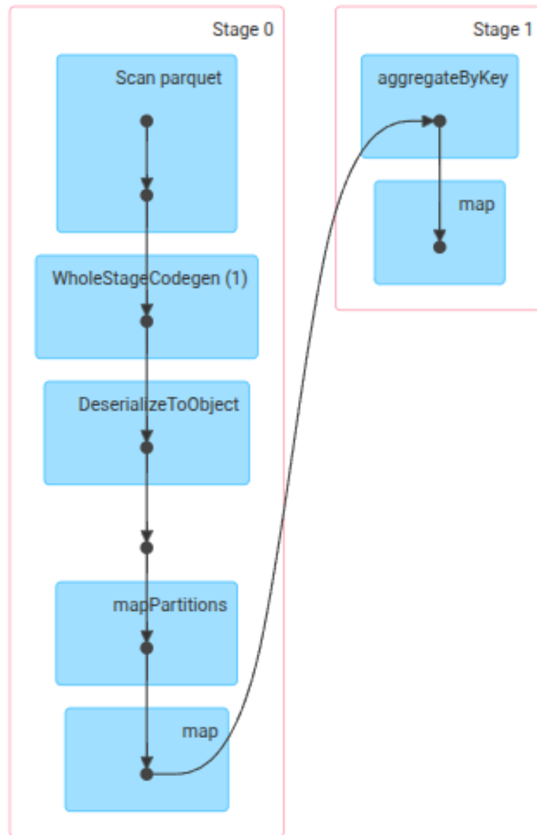
Figura 4. DAG di Spark per la Query 1: evidenzia la fase di aggregateByKey e la successiva trasformazione finale.
