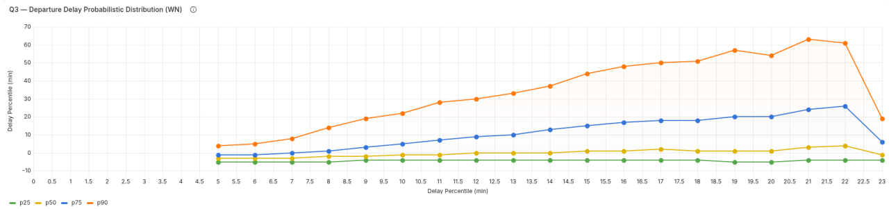
Figura 22. Risultati Query 3 (WN): Trend orario dei percentili di ritardo critici.
