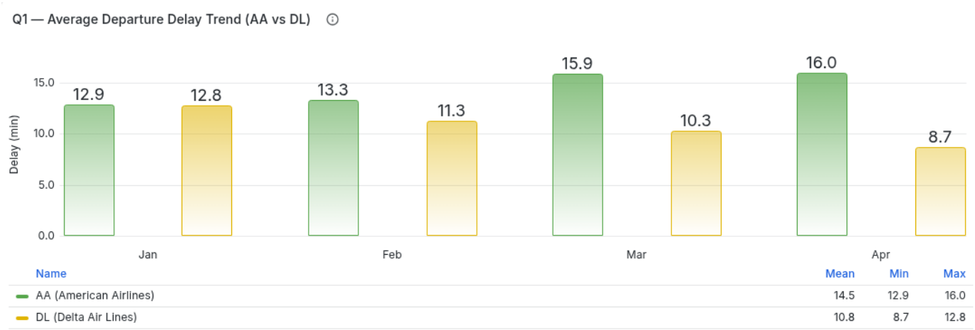
Figura 15. Risultati Query 1: Trend dei ritardi medi mensili.
