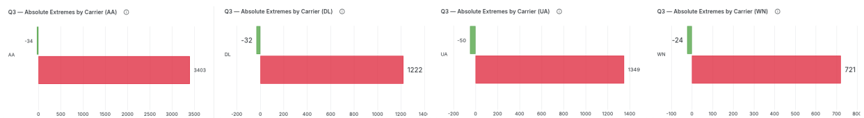
Figura 27. Risultati Query 3: Valori estremi dei ritardi per American Airlines (AA), Delta Air Lines (DL), United Airlines (UA) e Southwest Airlines (WN) (da sinistra a destra).
