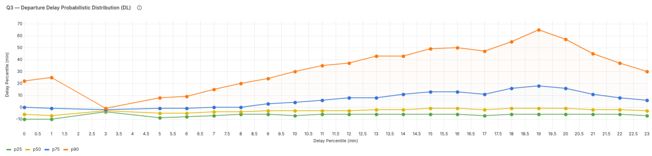
Figura 20. Risultati Query 3 (DL): Trend orario dei percentili di ritardo critici.
