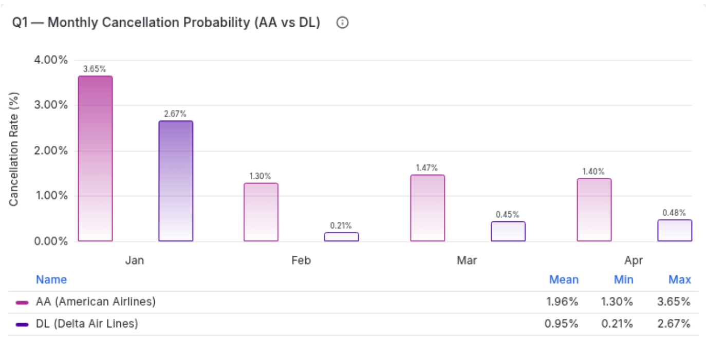
Figura 16. Risultati Query 1: Tasso e probabilità di cancellazione.
