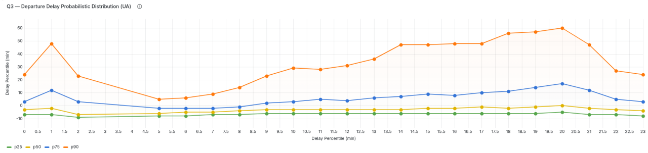
Figura 21. Risultati Query 3 (UA): Trend orario dei percentili di ritardo critici.
