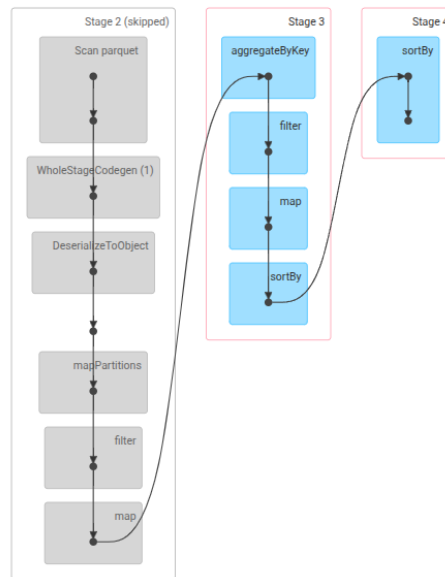
Figura 5. DAG di Spark per la Query 2: i tre job mostrano rispettivamente il filtraggio/aggregazione, il calcolo delle medie e l'ordinamento per il ranking top-10.
