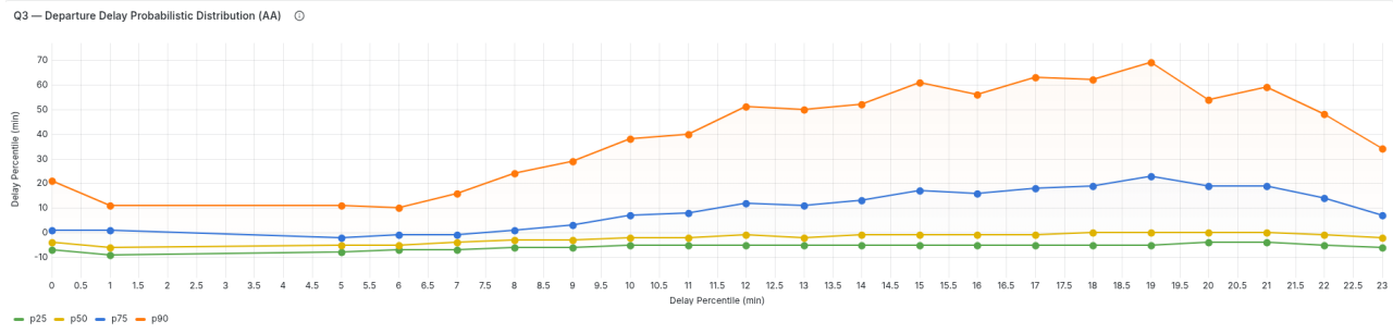
Figura 19. Risultati Query 3 (AA): Trend orario dei percentili di ritardo critici.
