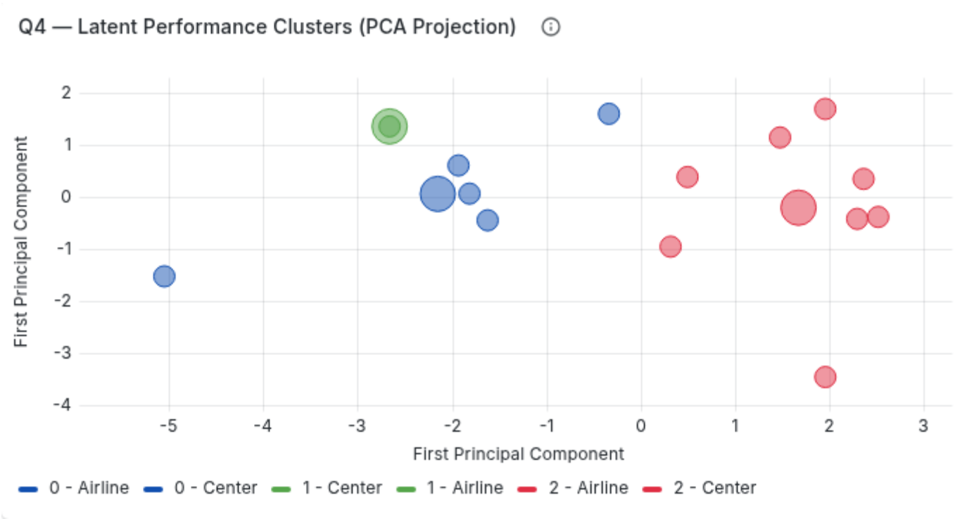
Figura 27. Risultati Query 4: Distribuzione geometrica dei cluster estratti tramite PCA.
