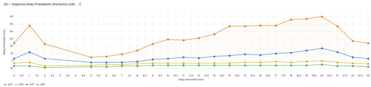
Figura 20. Risultati Query 3 (UA): Trend orario dei percentili di ritardo critici.
