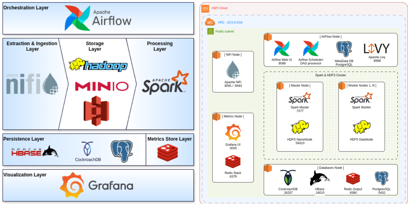
Figura 5. Diagrammi di Deployment e Big Data Stack. Il primo illustra i livelli logici del Big Data Stack utilizzato da SAE, mentre il secondo diagramma mostra la distribuzione dei componenti su AWS EC2 e EMR, .
