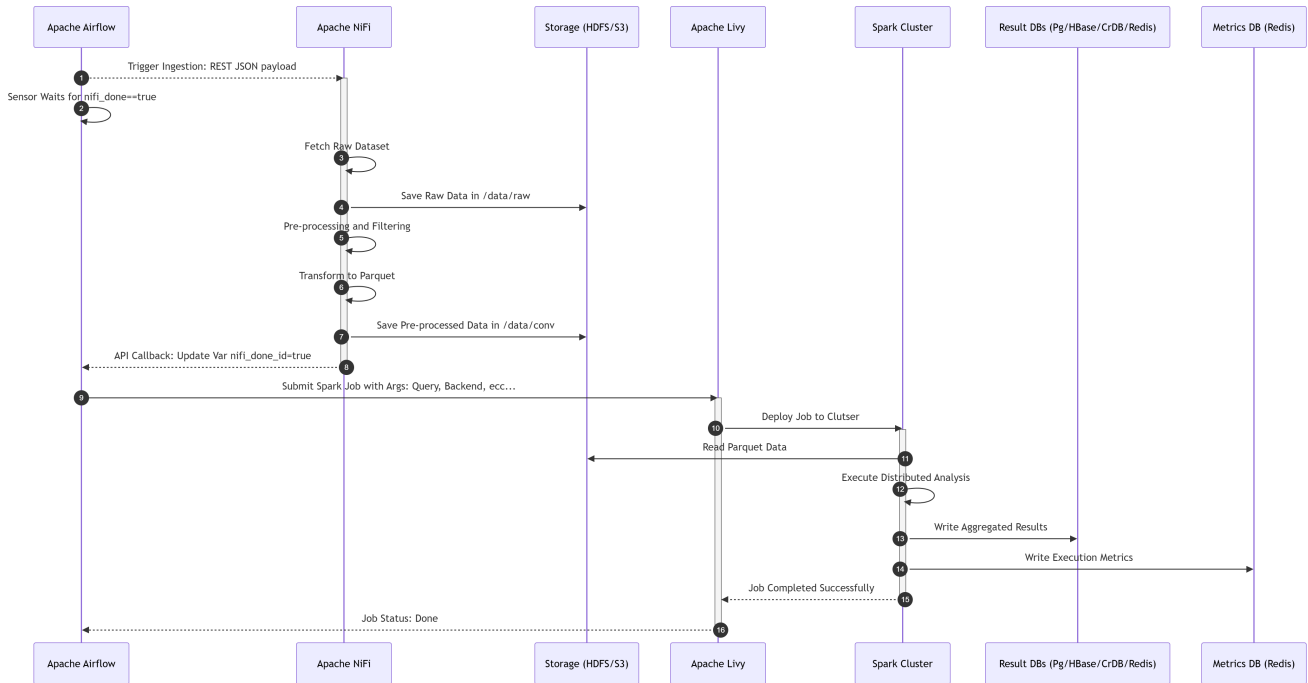
Figura 4. Diagramma di Sequenza di Sky Analytics Engine. Il diagramma illustra i componenti principali e i flussi di dati e controllo tra di essi durante l'esecuzione.
