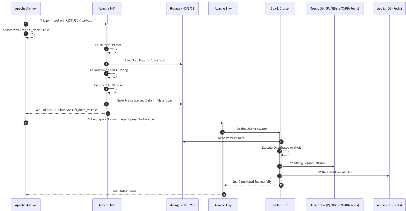
Figura 5. Diagramma di Sequenza di Sky Analytics Engine. Il diagramma illustra i componenti principali e i flussi di dati e controllo tra di essi durante l'esecuzione.
