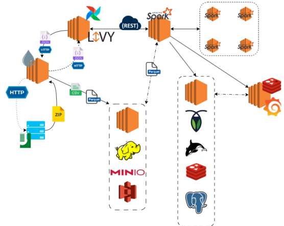
Vista Dinamica: Flusso di interazione dei componenti
