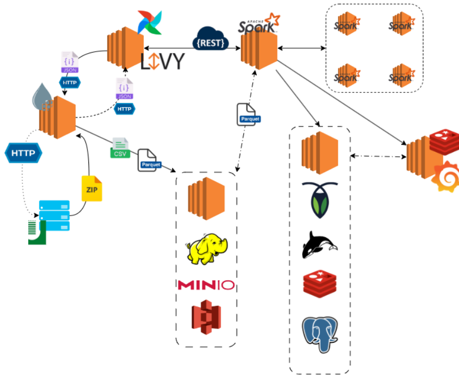
Figura 3. Il diagramma di interazione mostra le componenti chiave di SAE e le loro interazioni durante l'esecuzione di un job Spark, dall'ingestione dei dati alla persistenza dei risultati.
