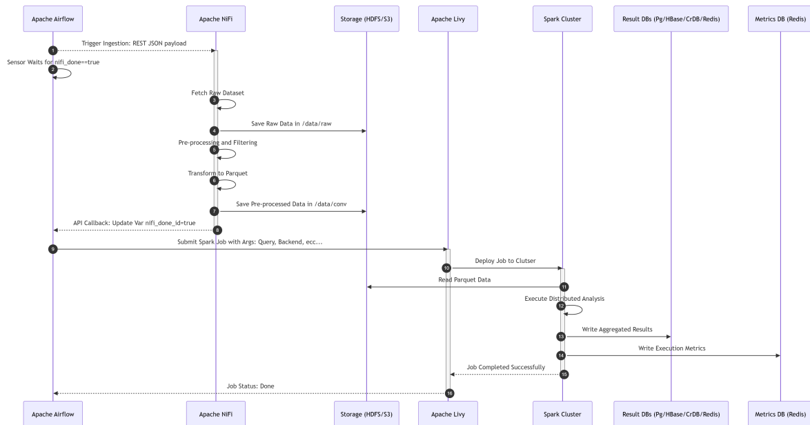
Figura 4. Il diagramma di sequenza illustra la coreografia temporale delle chiamate API, l'ingestione asincrona e il ciclo di vita del job Spark all'interno della piattaforma.
