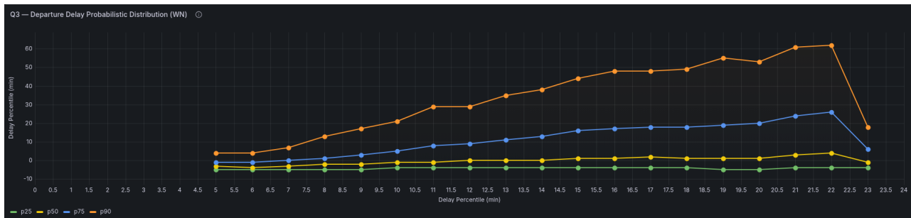
Figura 20. Risultati Query 3 (WN): Trend orario dei percentili di ritardo critici.
