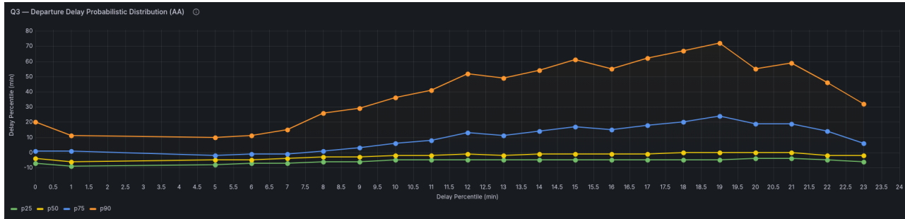
Figura 17. Risultati Query 3 (AA): Trend orario dei percentili di ritardo critici.
