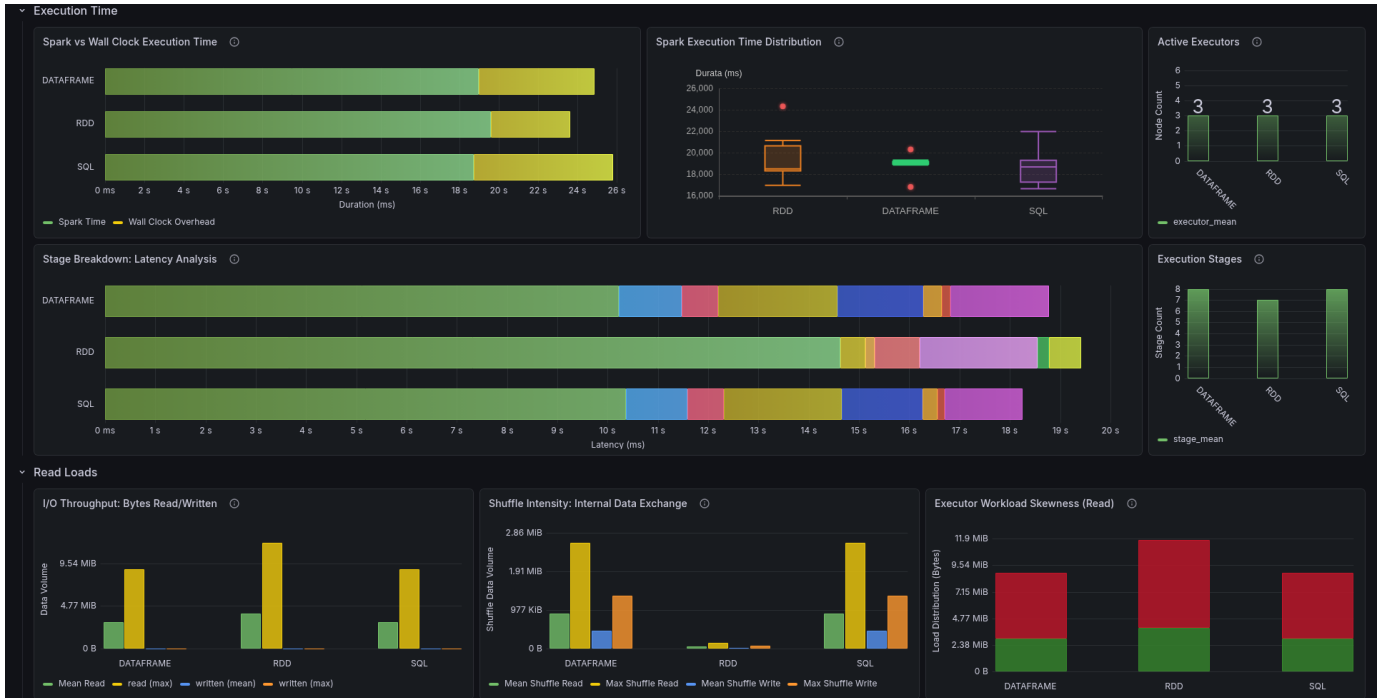
Figura 9. Telemetria Query 3 - Dettaglio Tempi AWS EC2 Standalone.
