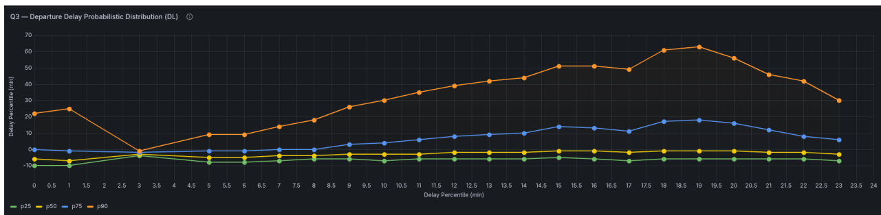
Figura 18. Risultati Query 3 (DL): Trend orario dei percentili di ritardo critici.
