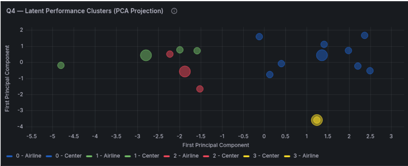
Figura 26. Risultati Query 4: Distribuzione geometrica dei cluster estratti tramite PCA.
