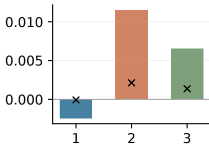
Diferença de W_{90}
