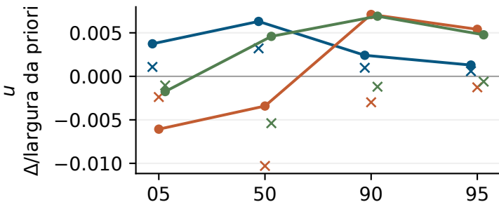
Diferença de quantis
