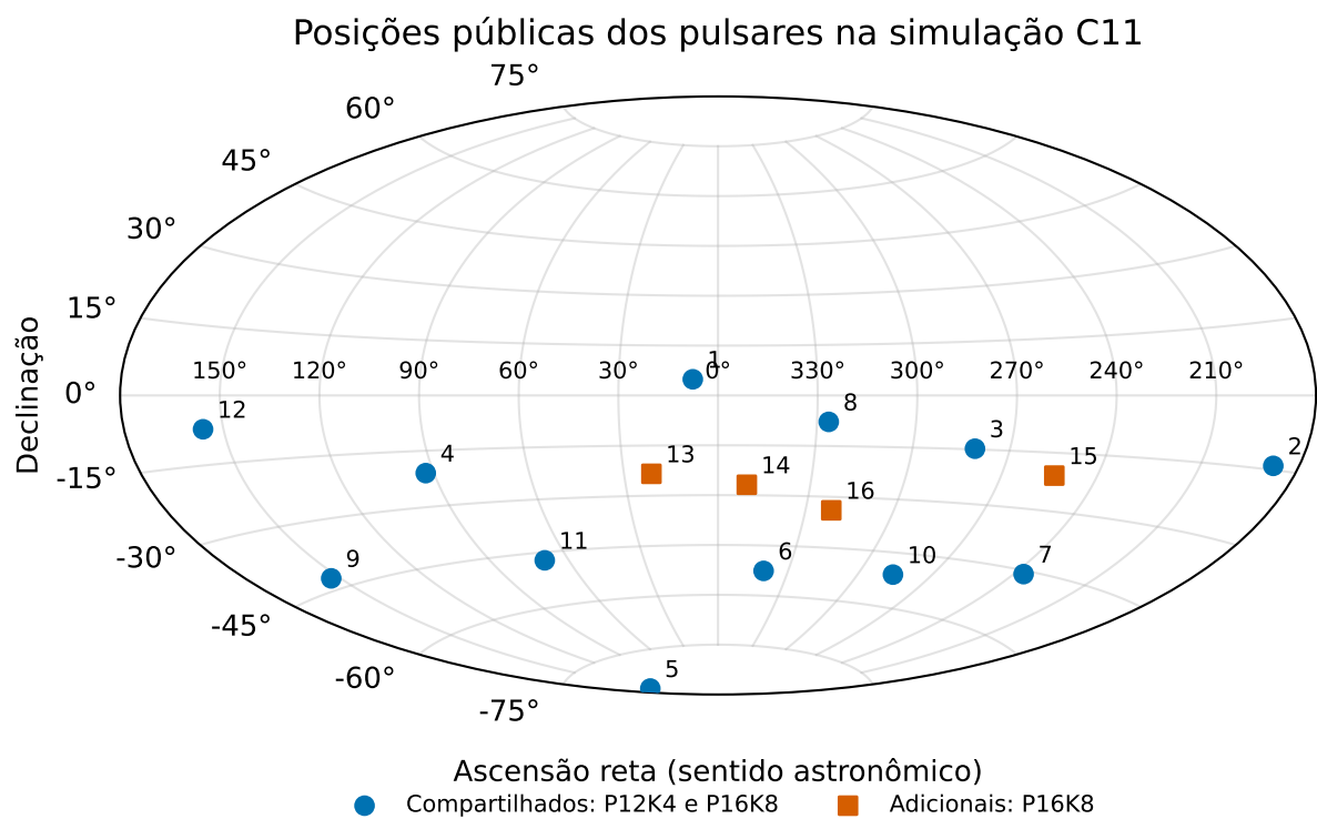
FIGURA 10.1 – Direções públicas dos 16 pulsares selecionados do produto MeerKAT, com os 12 compartilhados por P12K4 e P16K8 e os quatro adicionais de P16K8. Os números correspondem à ordem determinística de seleção registrada nos metadados. Apenas as posições são observacionais: distâncias, sinais e ruídos usados no experimento são sintéticos. Fonte: metadados MeerKAT, DOI 10.57891/j0vh-5g31, CC BY 4.0; figura produzida neste trabalho.
