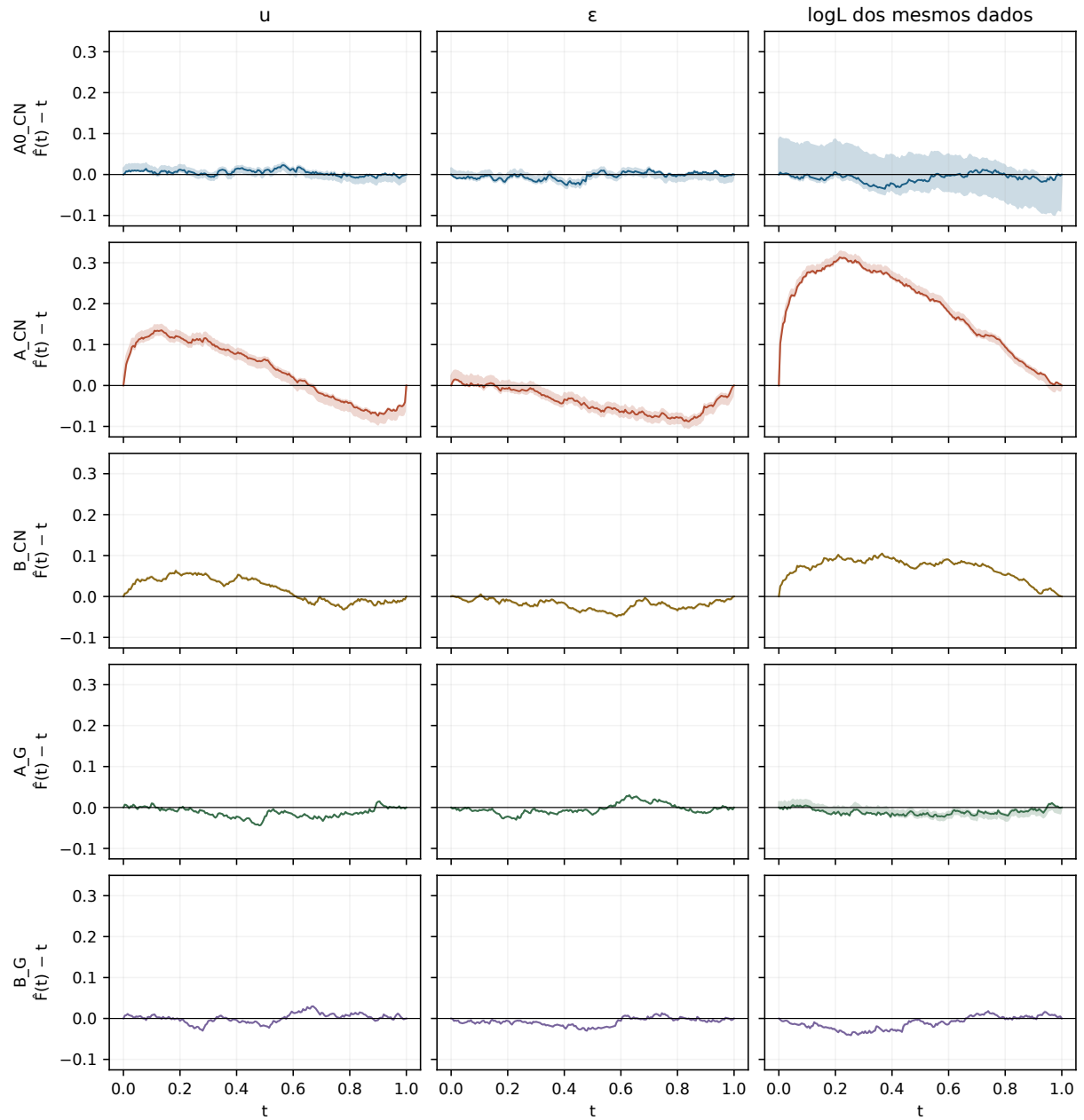
FIGURA 9.1 – Desvios das CDFs empíricas dos PITs em relação à uniforme. Linhas: representação nominal; faixas: envelope das CDFs permitido pelos intervalos numéricos, incluindo os casos [0, 1] . Cada painel usa todos os 500 dados da priori conjunta. A interpretação dos testes é dada pela Tabela 9.2, com as correções de multiplicidade.
