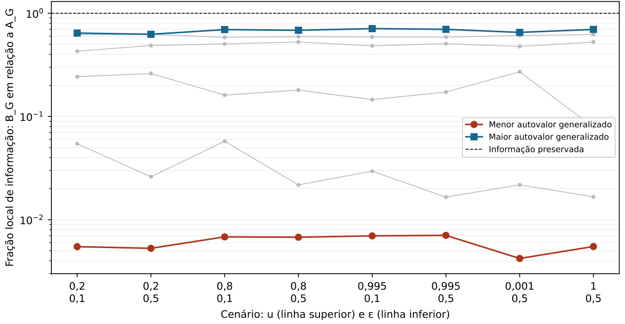
FIGURA 9.4 – Autovalores generalizados de I_{B\_G}v = \lambda I_{A\_G}v nos oito cenários. As curvas cinzas mostram os quatro autovalores intermediários. A comparação é entre o experimento normal por frequência e sua compressão linear, com seis coordenadas e geometria fixas; não é uma comparação de evidências ou de A0_CN com uma lei aproximada.
