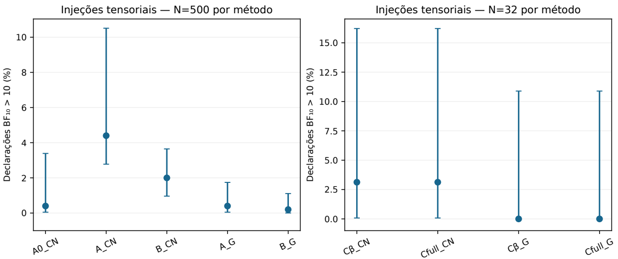
FIGURA 9.2 – Falsos positivos no limiar BF_{10} > 10 . Pontos: taxas nominais; barras: união dos intervalos binomiais a 95% considerando a sensibilidade numérica. Os painéis têm tamanhos amostrais e escalas verticais diferentes. O subconjunto C tem finalidade descritiva.
