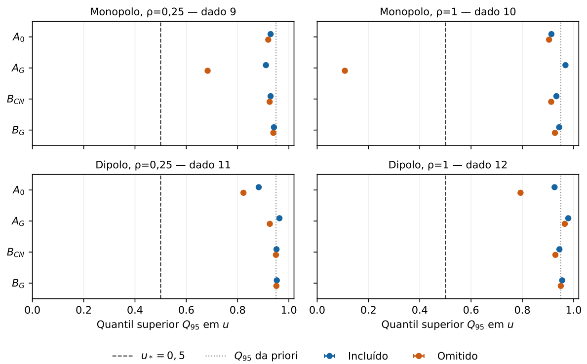
FIGURA 8.3 – Quantis superiores nos quatro casos fixos com contaminantes. Cada comparação inclusão/omissão usa a mesma observação dentro da família analisada; os controles gaussianos não são a mesma observação das estatísticas CN. As barras representam intervalos numéricos, frequentemente menores que os símbolos, e não intervalos populacionais. As linhas indicam a massa injetada e o quantil da priori uniforme. Não se estima cobertura com esses quatro casos de engenharia.
