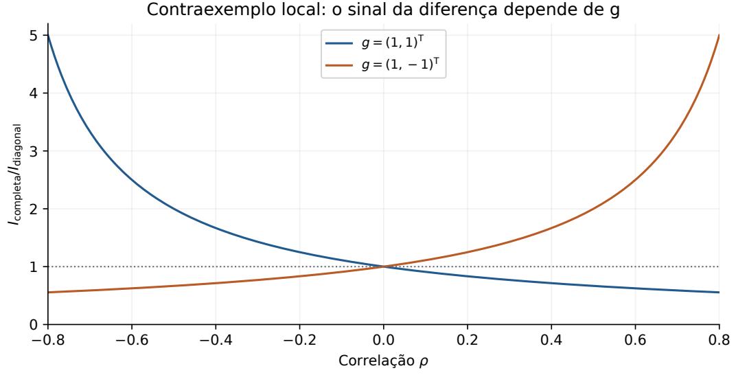
FIGURA 8.2 – Razão analítica entre as informações de Fisher completa e diagonal no exemplo de duas dimensões. A mesma correlação pode aumentar ou diminuir essa razão, conforme a derivada da média g . Trata-se de um contraexemplo local, não de uma previsão quantitativa dos limites PTA.
