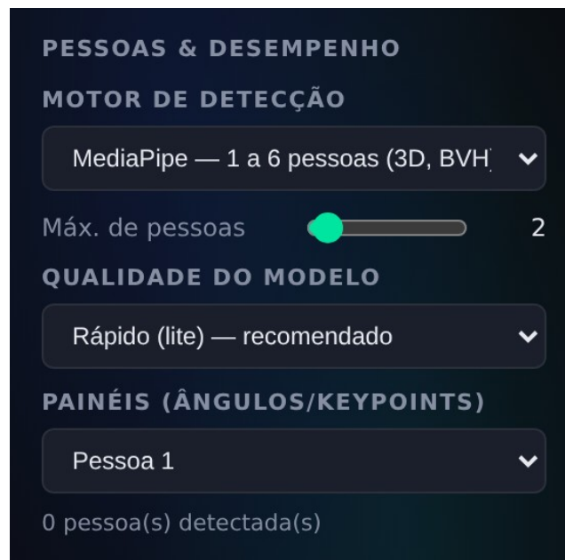
Figura 7 — Painel Pessoas & desempenho: motor de detecção, quantidade de pessoas e qualidade.
