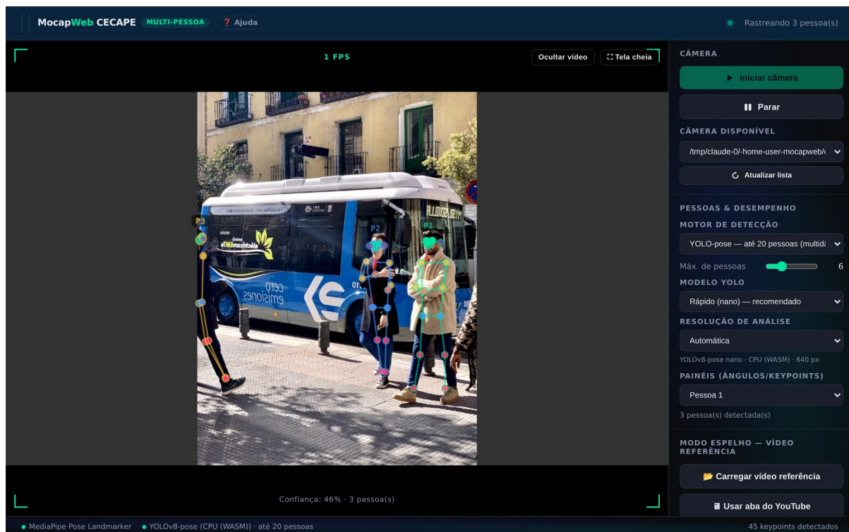
Figura 6 — Sistema rastreando 3 pessoas (detecção real sobre uma foto de teste): cada pessoa com sua cor e etiqueta P1, P2, P3.
