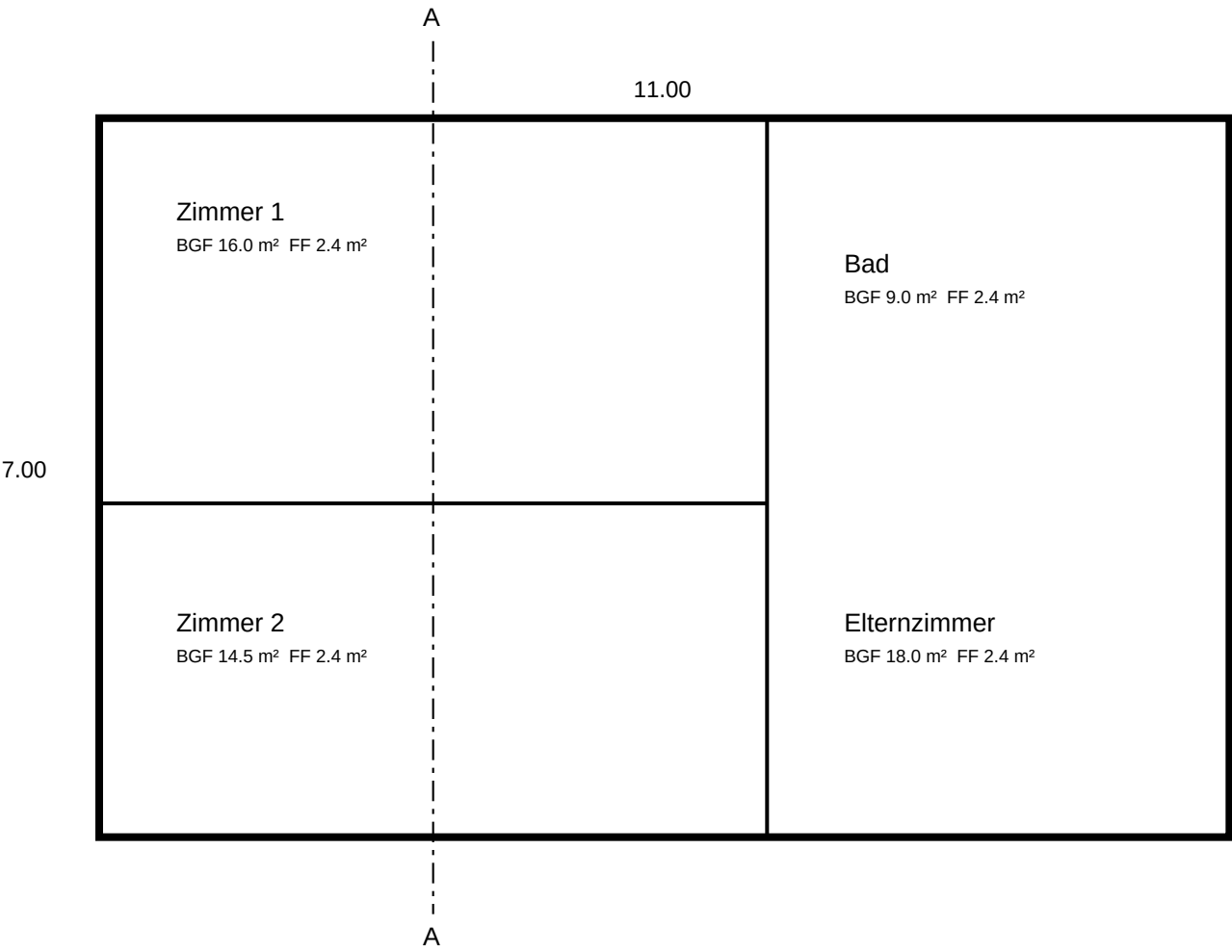
Grundriss OG, OK FFB +2.80 Fensterflächen gemäss Raumstempel, Wandstärke Aussenwand 36 cm
