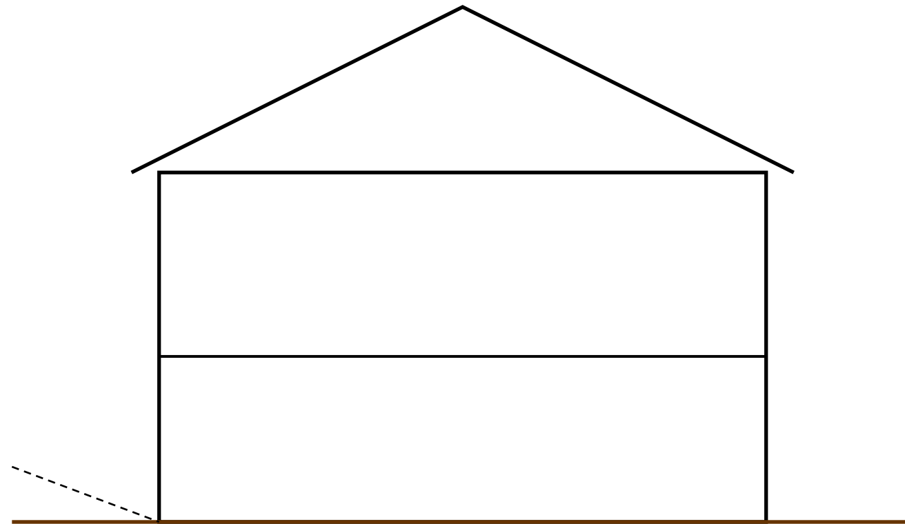
Schnitt A-A Geschosshöhen 2.60 m, UK Fundament 453.20 m ü. M., Terrain gestrichelt Aufbau Dach: Ziegel, Lattung, Unterdach, Sparren; Decke Stahlbeton 22 cm
