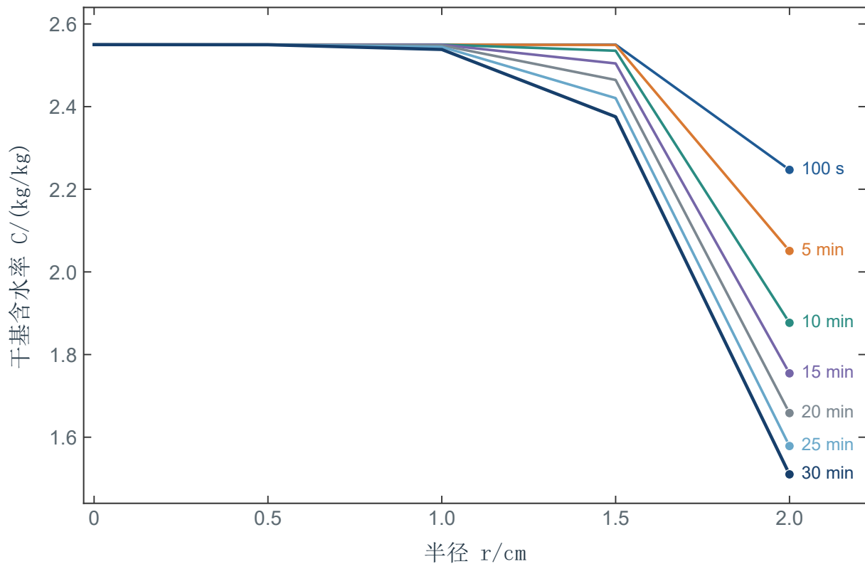
图 1：不同时刻的径向含水率分布
