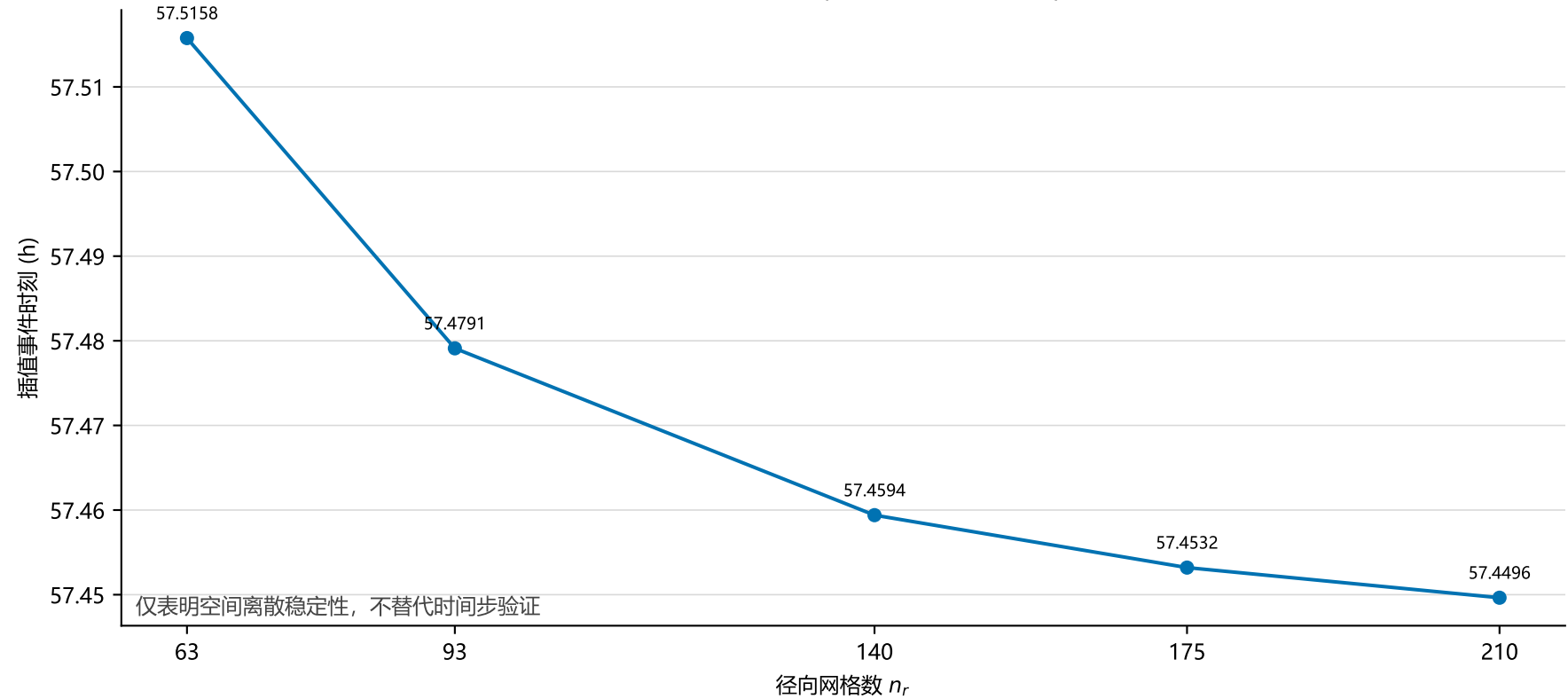
Q3 空间网格收敛 (五组网格, dt=60 s)
