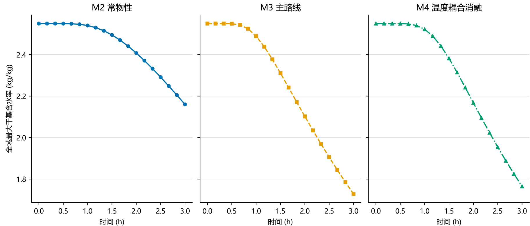
三个模型在不同时间的最大含水率轨迹
