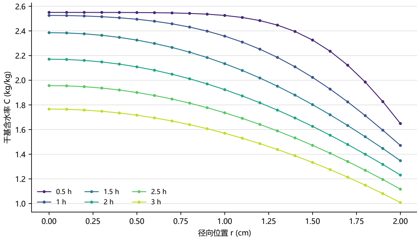
问题二：内部温度场下的含水率径向剖面
