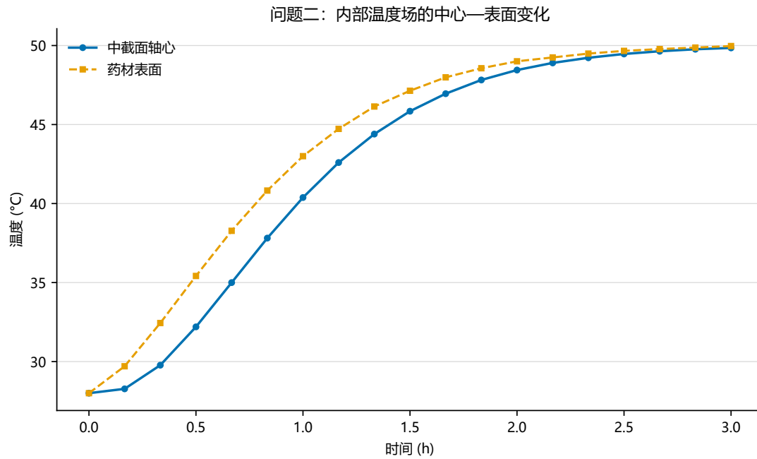
图 3 问题二内部温度场的中心—表面轨迹
