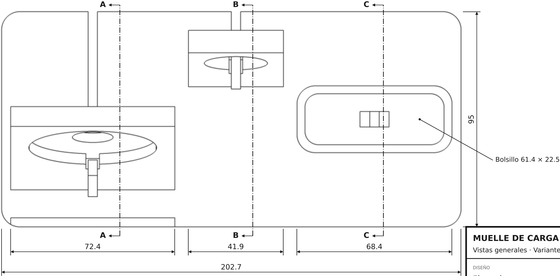
PLANTA (SUPERIOR)
