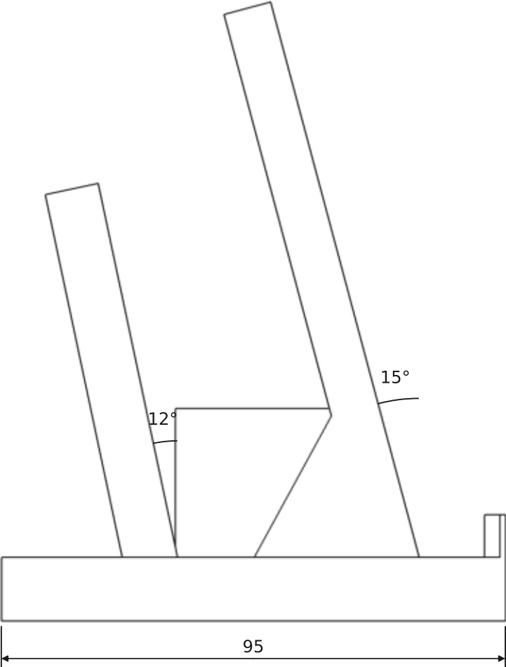
PERFIL IZQUIERDO
