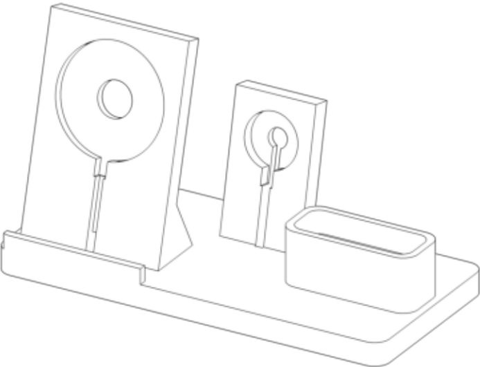
ISOMÉTRICA (escala 1:2.4)
