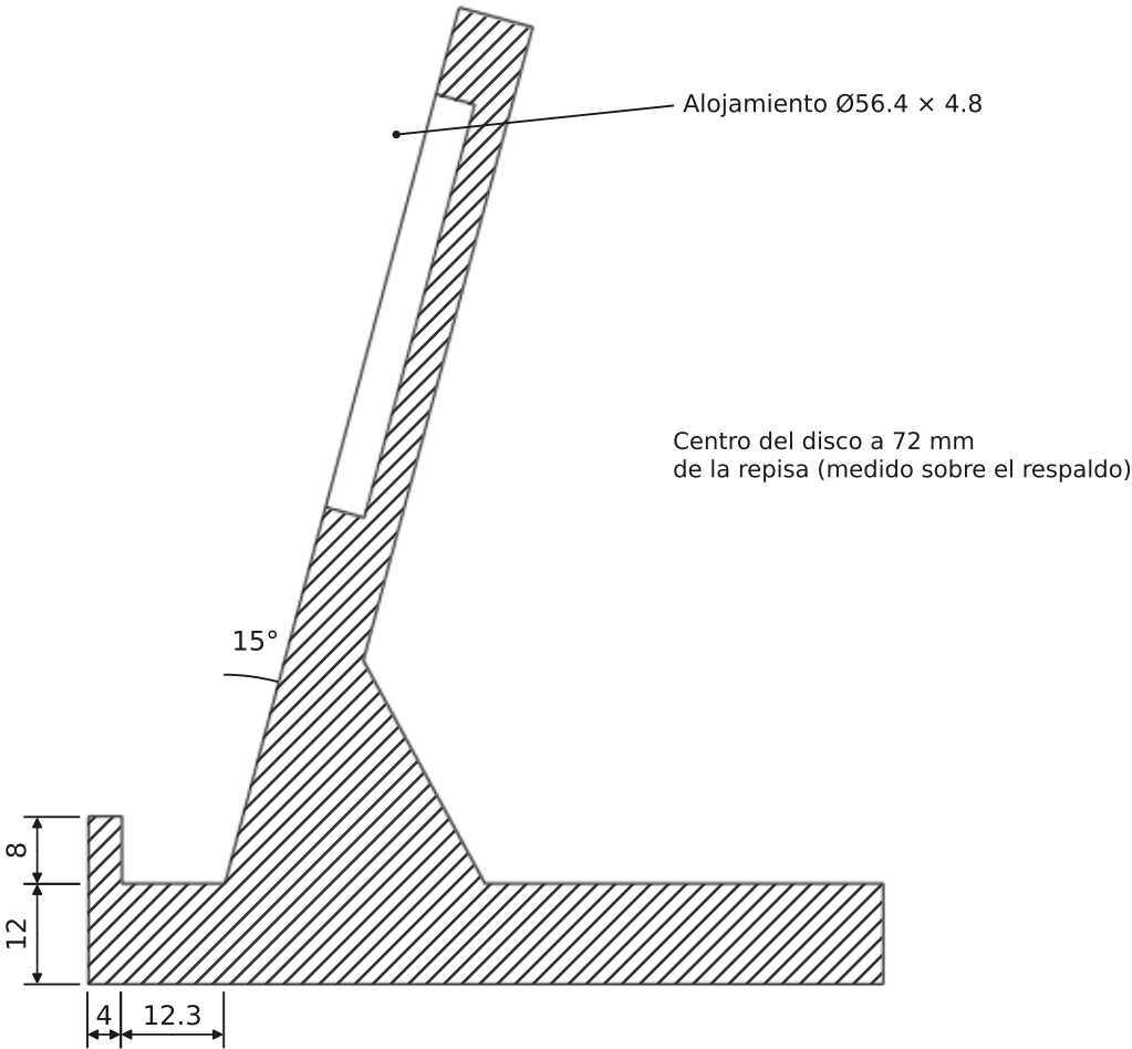
SECCIÓN A-A · CELULAR (MagSafe)
