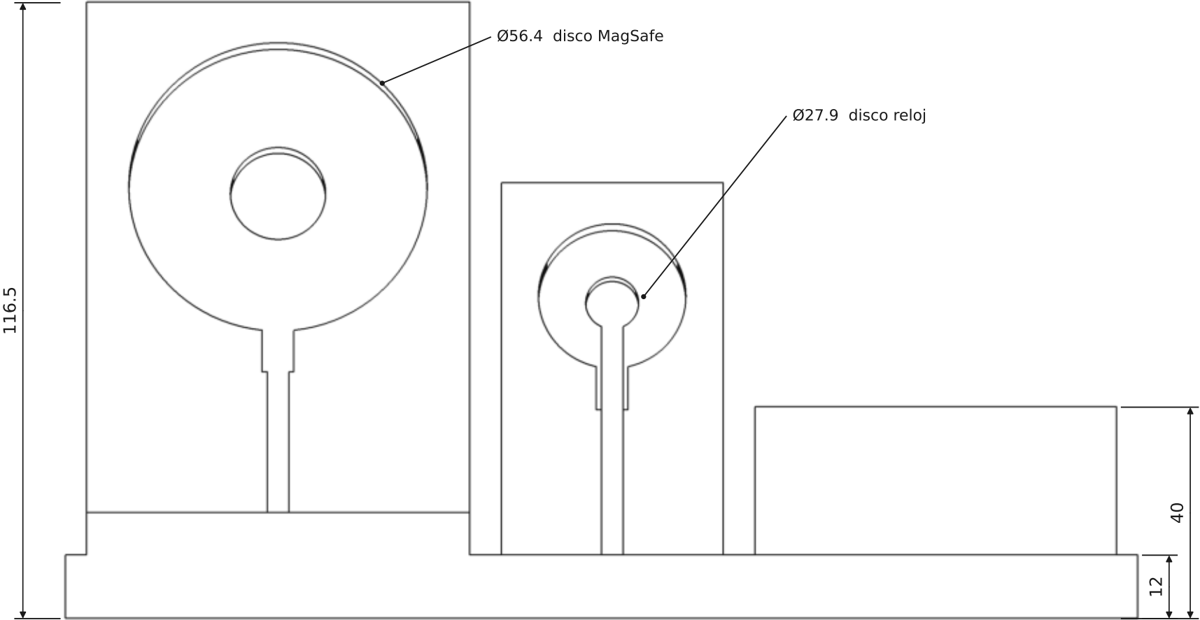
ALZADO (FRONTAL)
