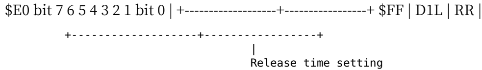
Fig. 30 D1L/RR (set per slot)
