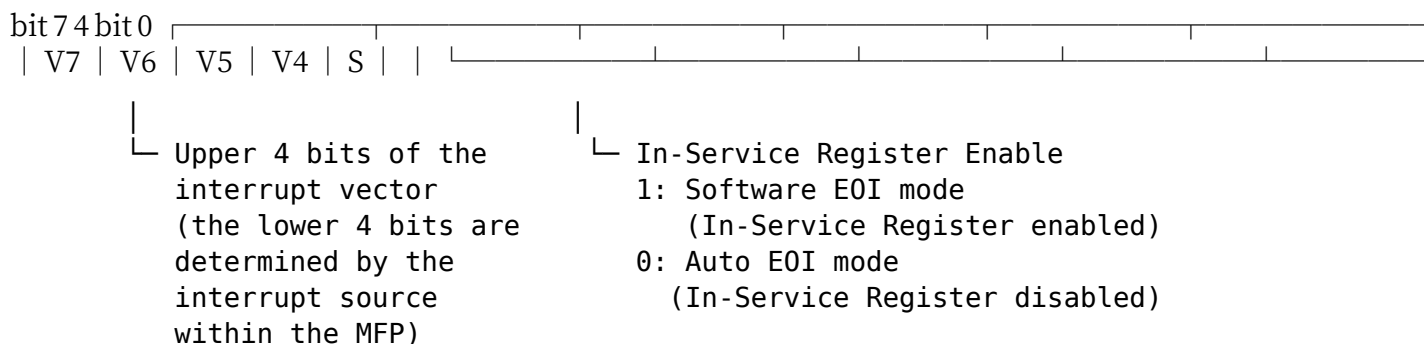
● Fig. 6 VR (Vector Register) $E88017
