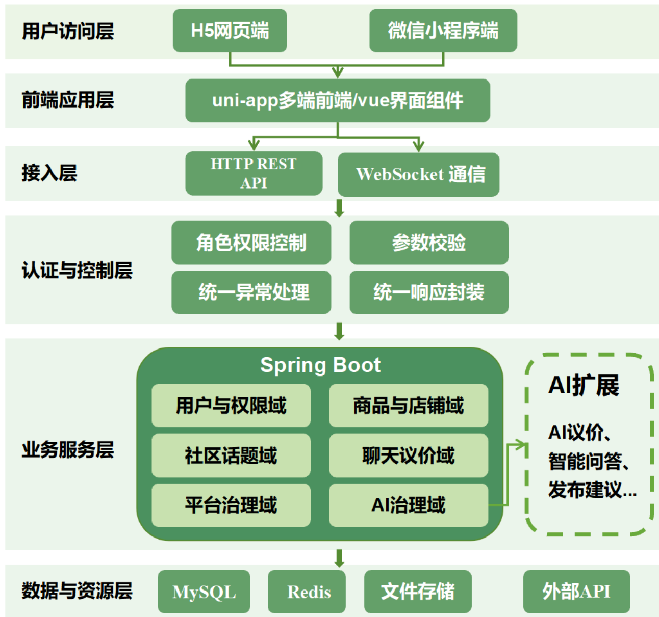
图 2-1 松果集市总体架构图
