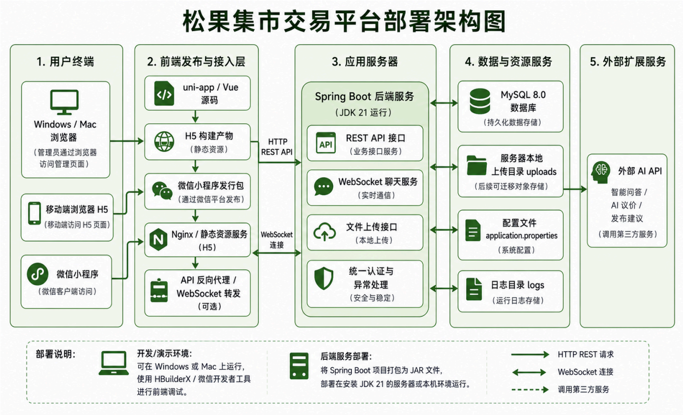
图 7-1 松果集市部署架构图
