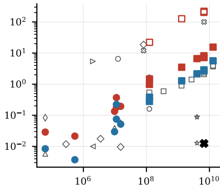
model parameters
