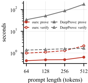
(a) GPT-2
