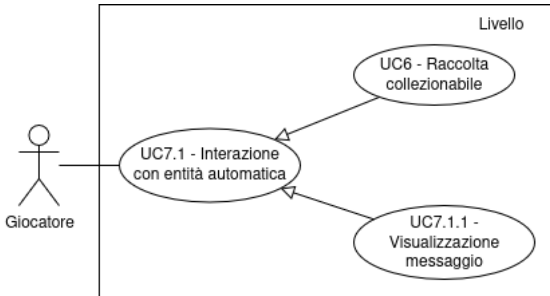
Figura 8: Interazione entità automatica
