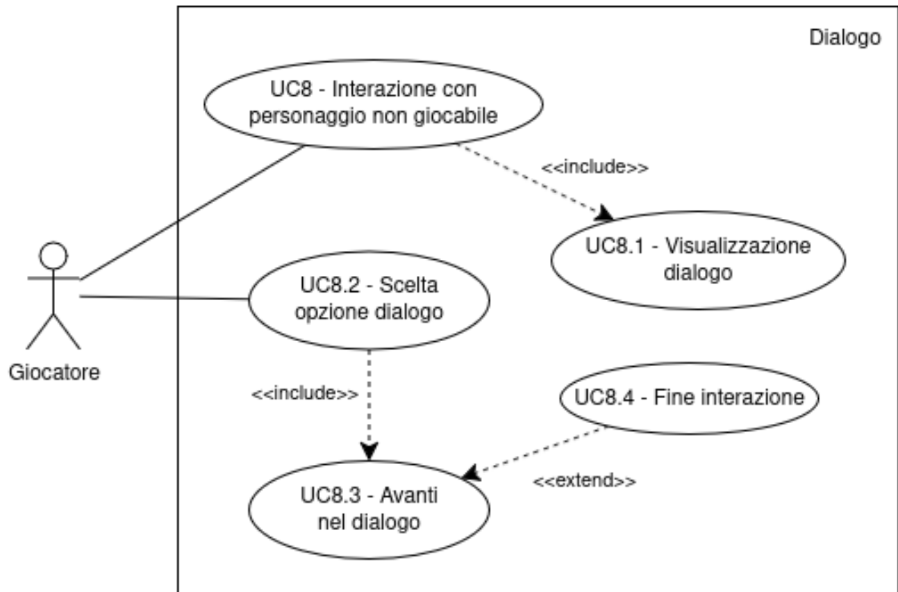
Figura 10: Interazione personaggio non giocabile
