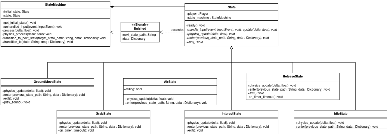
Figura 4: Diagramma sulla struttura della macchina di stati
