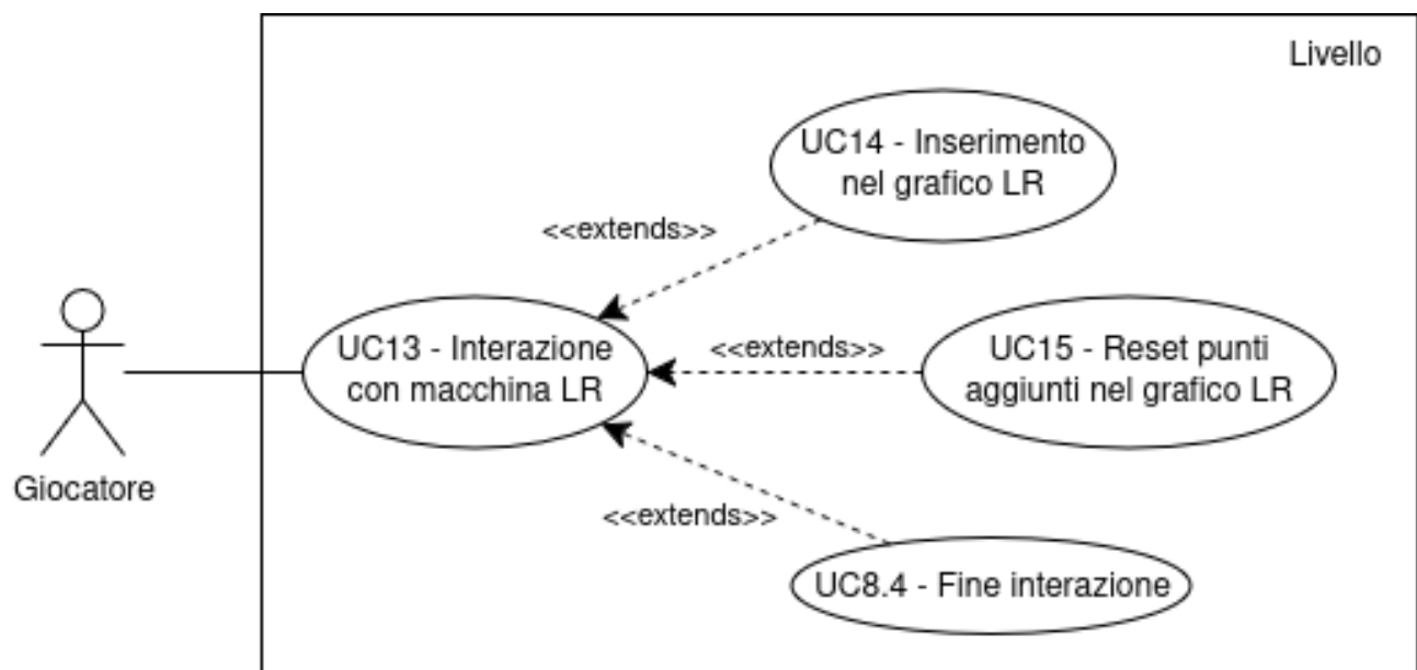
Figura 16: Interazione la macchina LR
