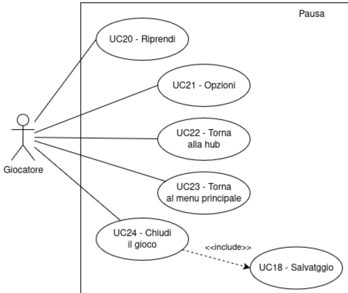
Figura 19: Menu di pausa
