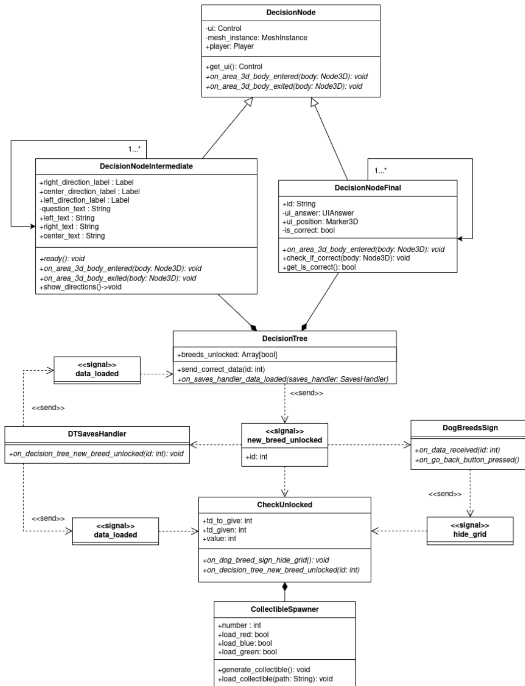
Figura 14: Diagramma sul funzionamento dell'Albero di decisione
