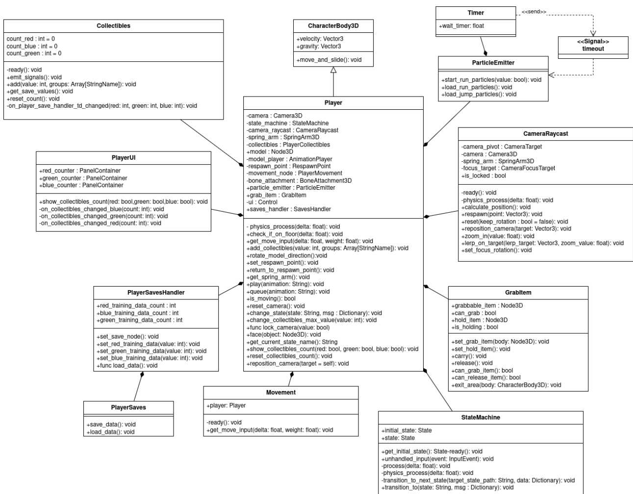
Figura 2: Diagramma delle classi del giocatore
