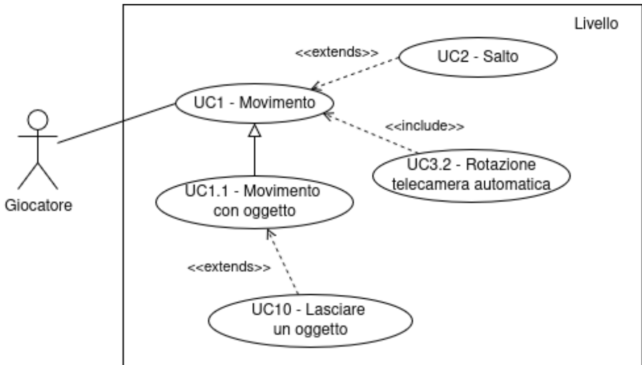
Figura 2: Movimento
