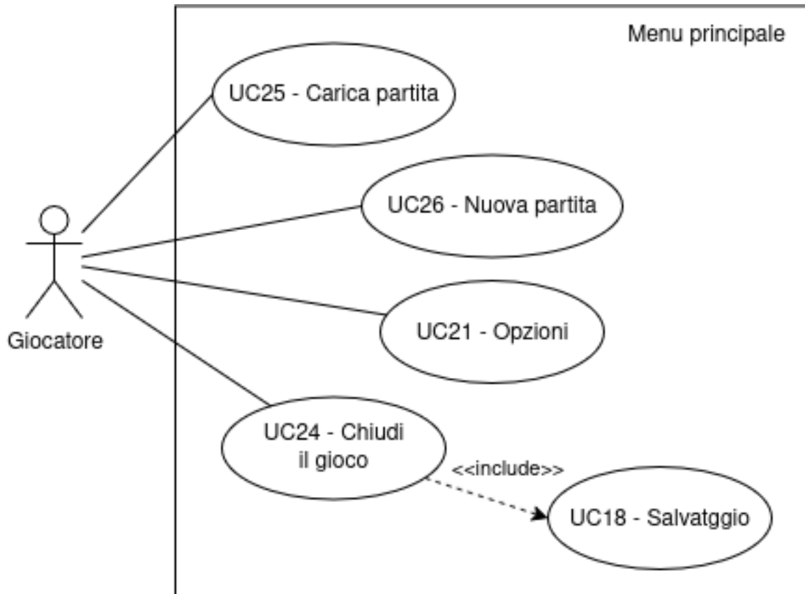
Figura 11: Menu principale
