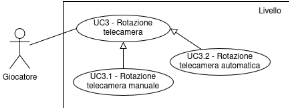
Figura 3: Rotazione telecamera
