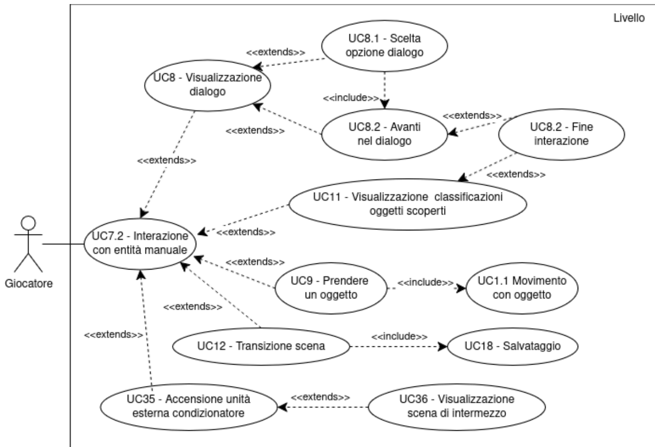
Figura 7: Interazione manuale
