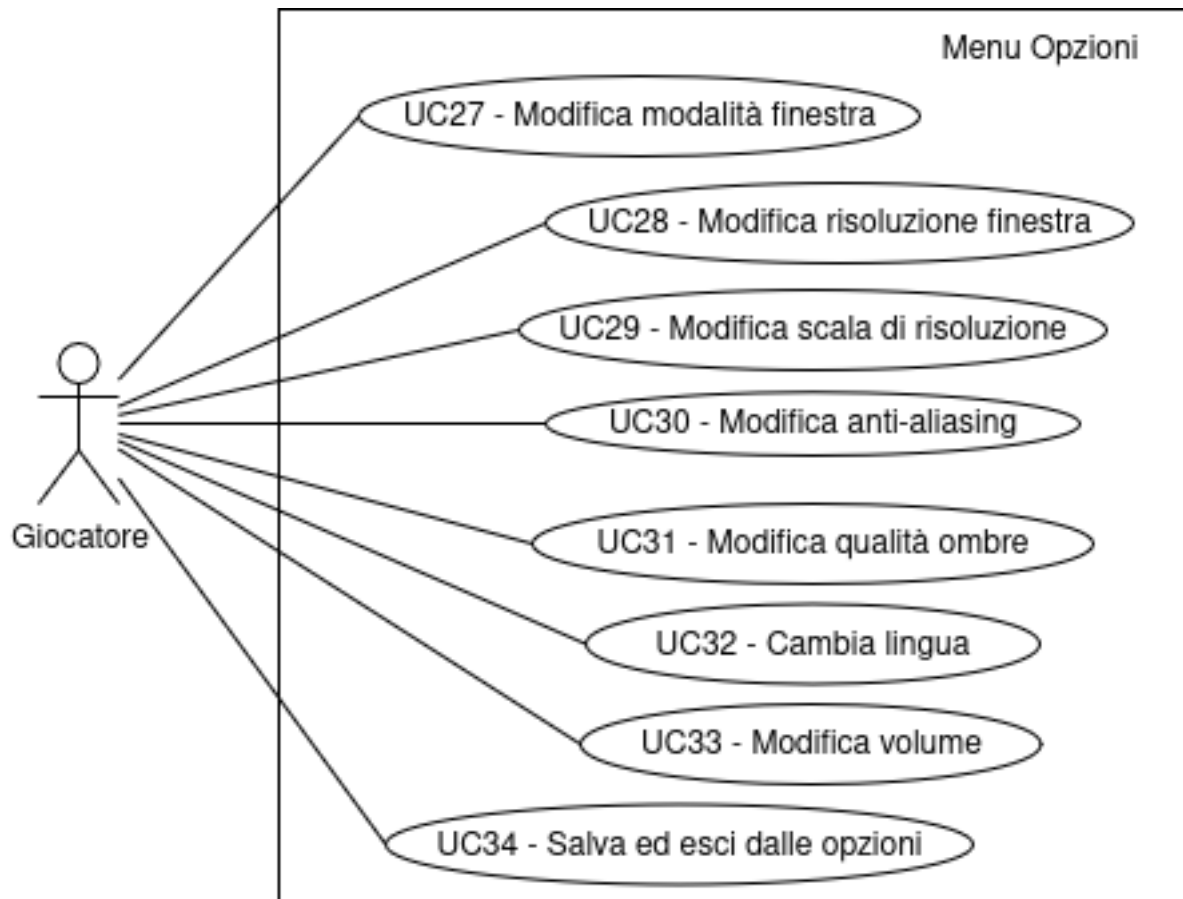
Figura 12: Menu opzioni
