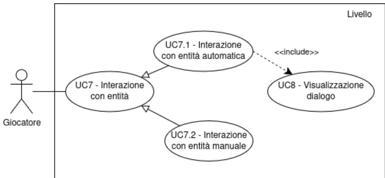
Figura 6: Interazione entità
