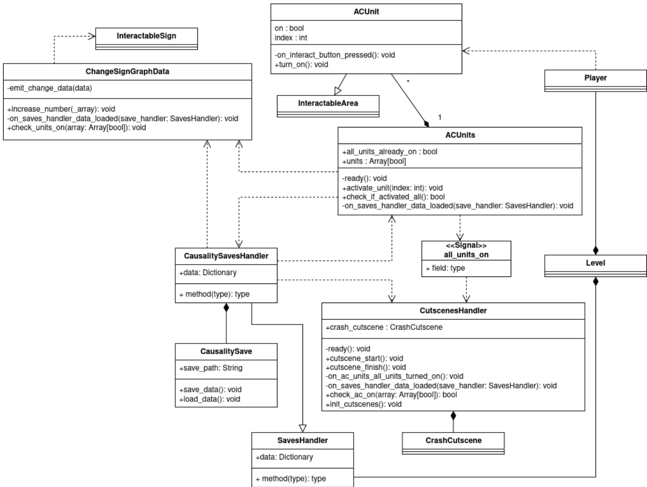
Figura 15: Diagramma del livello della causalità
