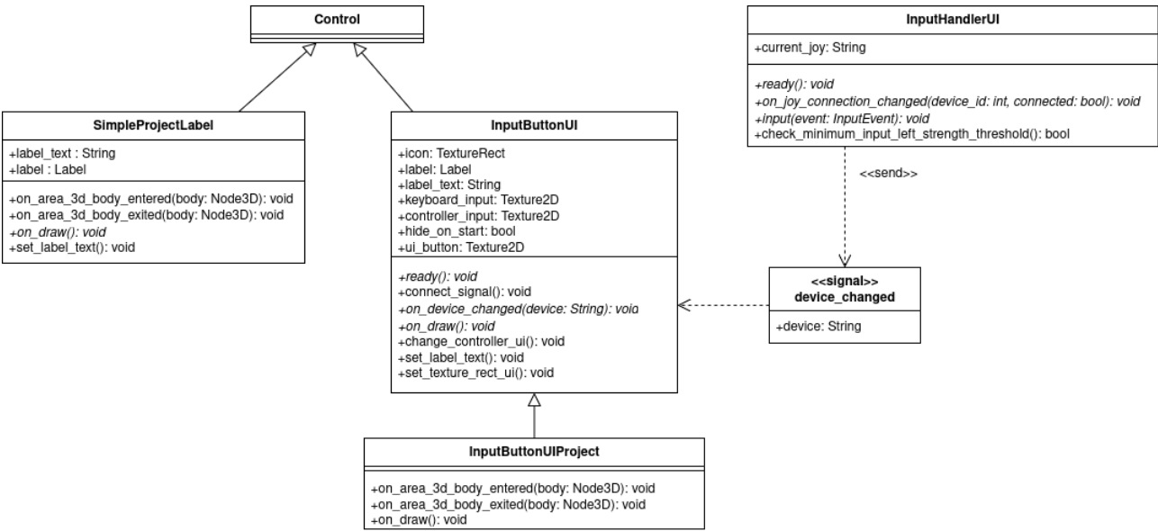
Figura 8: Diagramma dei vari tipi di UI
