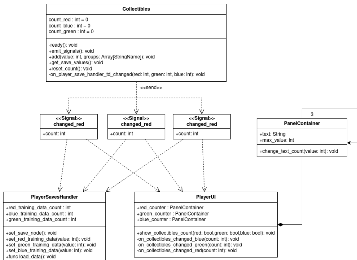
Figura 6: Diagramma delle classi della UI del giocatore
