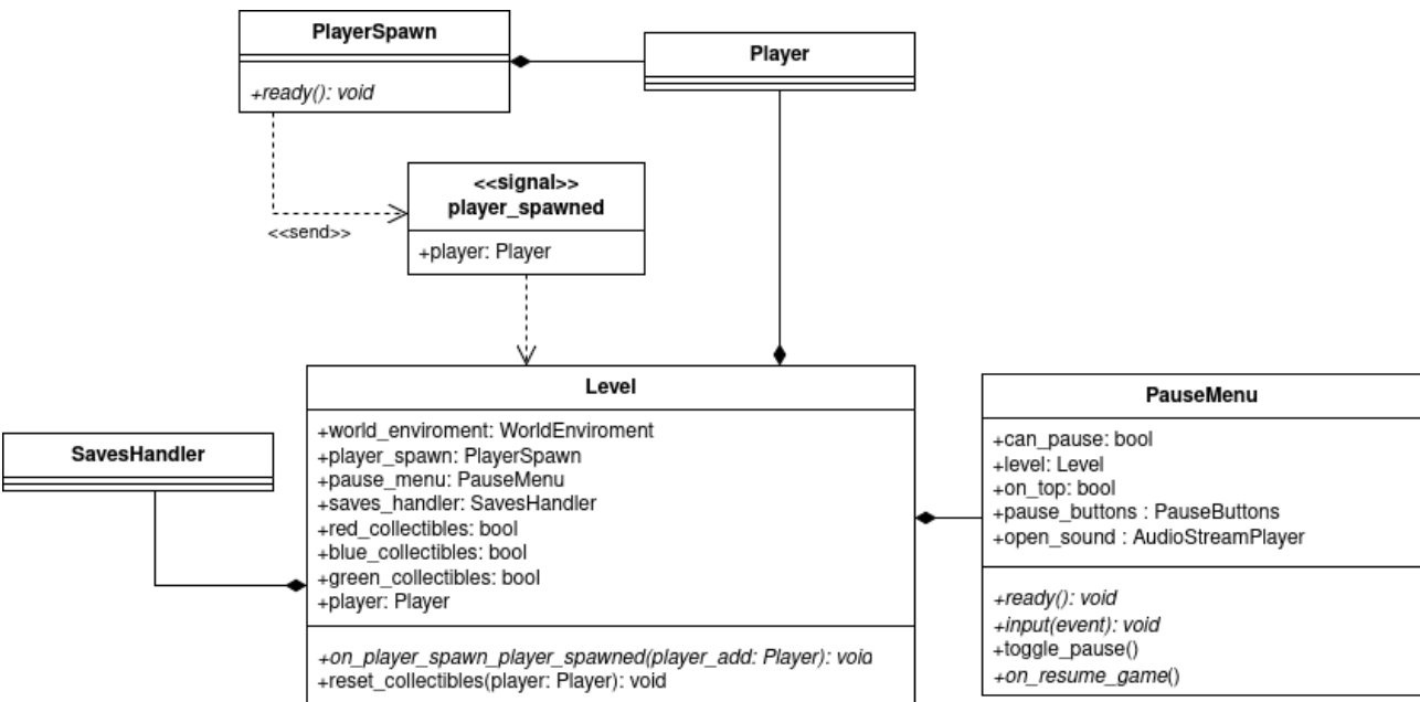
Figura 12: Diagramma di un livello base
