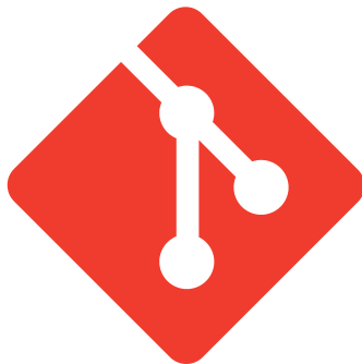
Git
