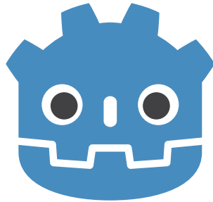
Godot
