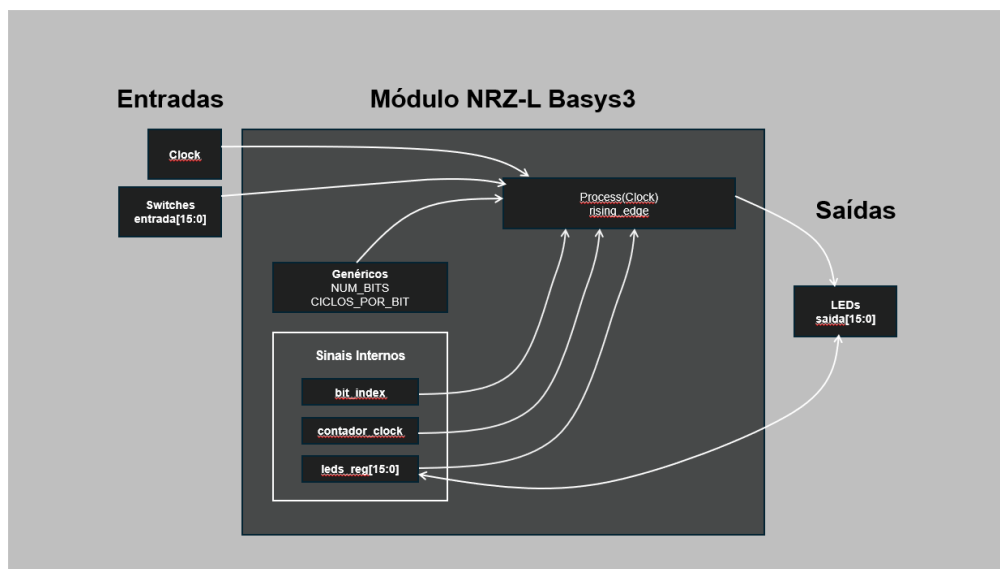
Figura 1 - Diagrama de blocos Módulo NRZ-L
