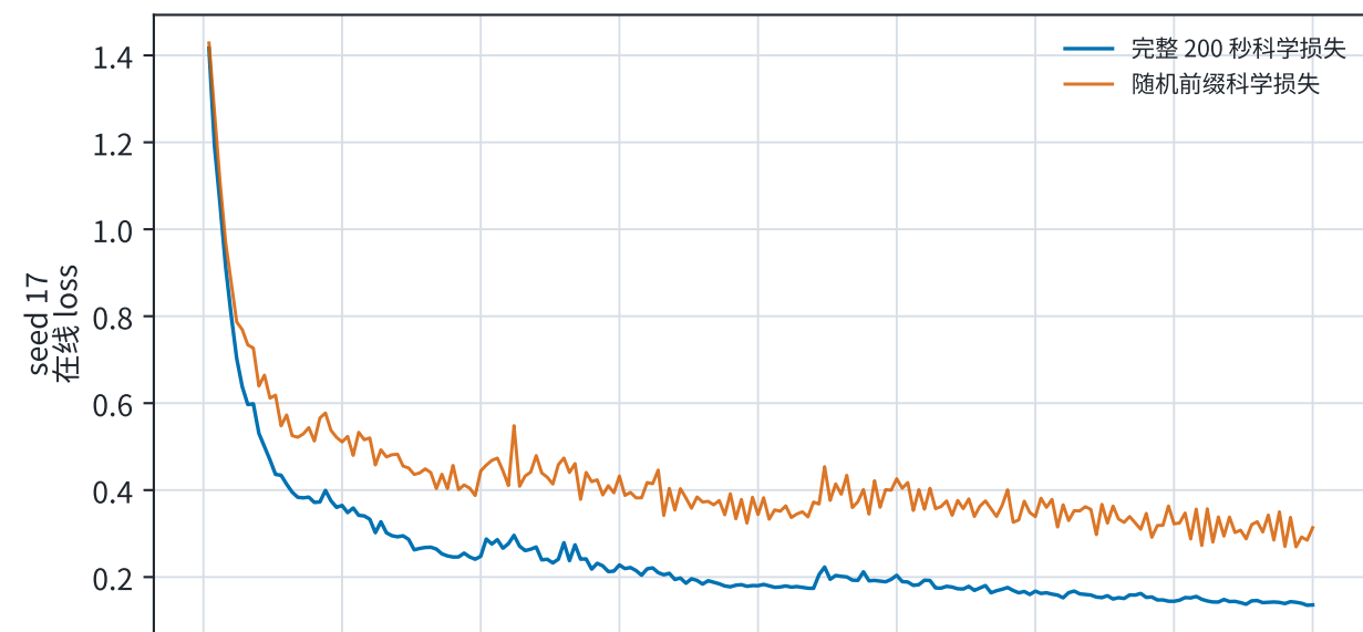
Phase48 联合从头训练：前缀任务学会了，但终点校准仍有代价
