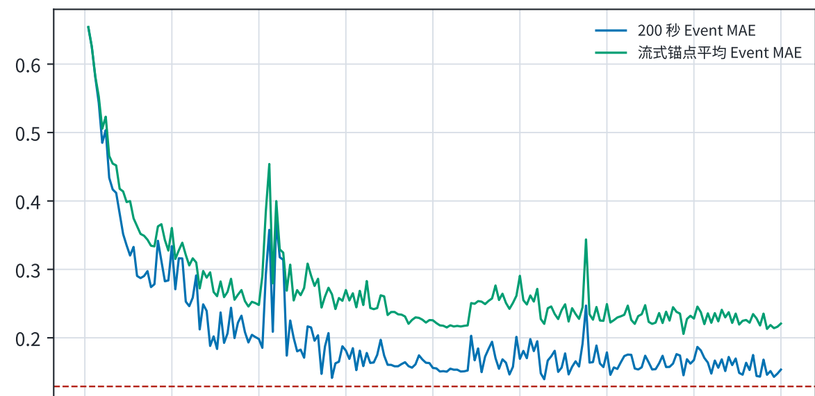
Phase48 联合从头训练：前缀任务学会了，但终点校准仍有代价
