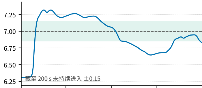
Samos 2020 M7.0 | 参考 7.0 | 200 s 预测 6.830
