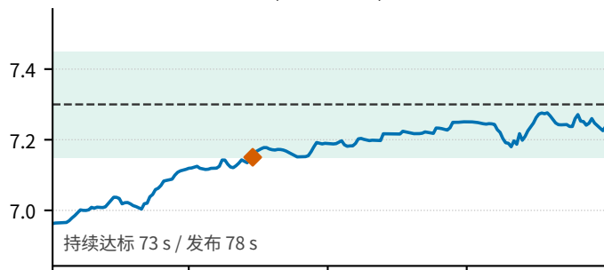
Sand 2025 M7.3 | 参考 7.3 | 200 s 预测 7.238
