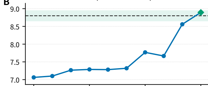
B Maule2010 | 目录 Mw 8.80 | n200=3
