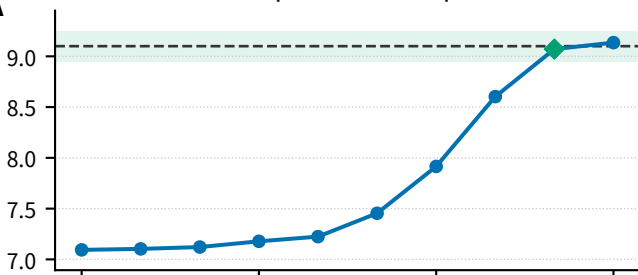
A Tohoku2011 | 目录 Mw 9.10 | n200=103
