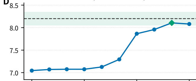
D Chignic2021 | 目录 Mw 8.20 | n200=6
