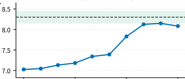
C Illapel2015 | 目录 Mw 8.30 | n200=4
