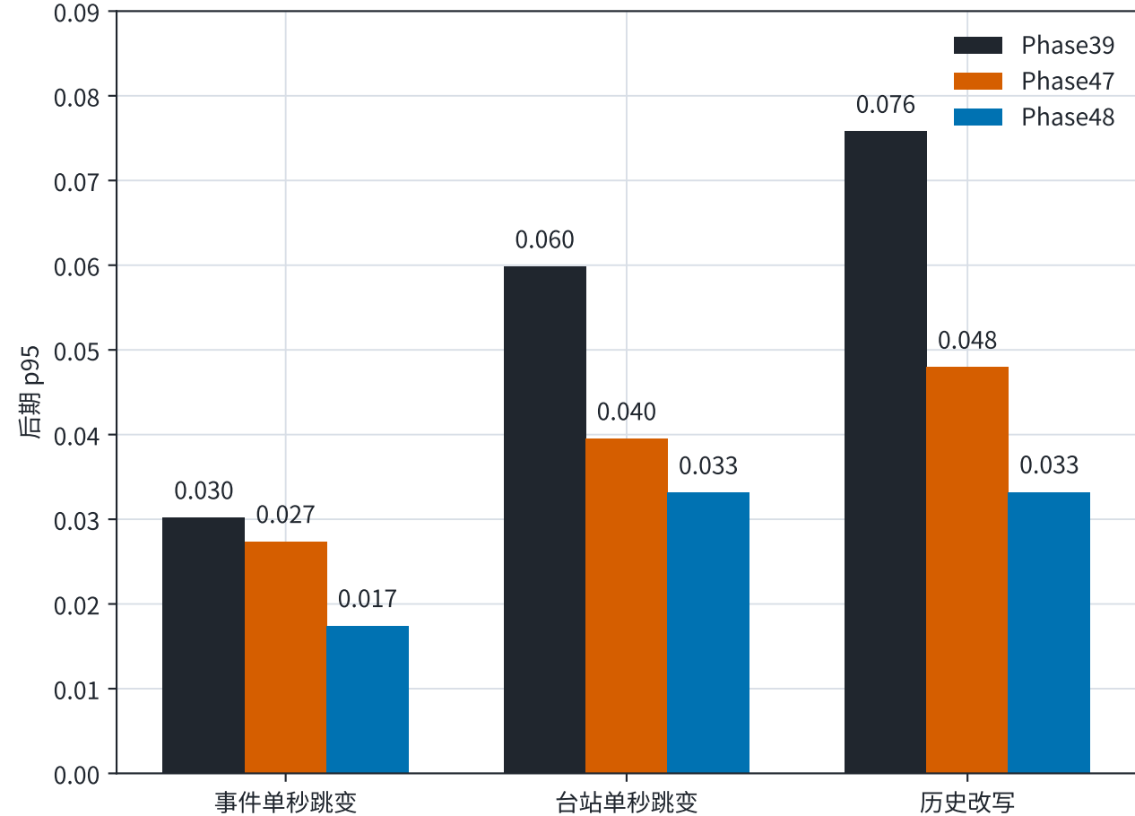
流式稳定性：Phase48 改善最明显
