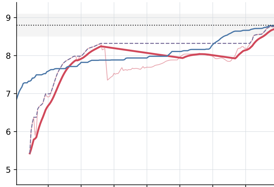
B. Maule2010 | Mw 8.80
