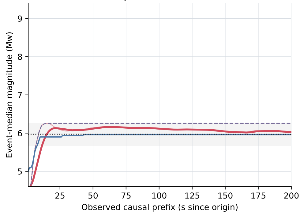
D. Parkfield2004 | Mw 5.97
