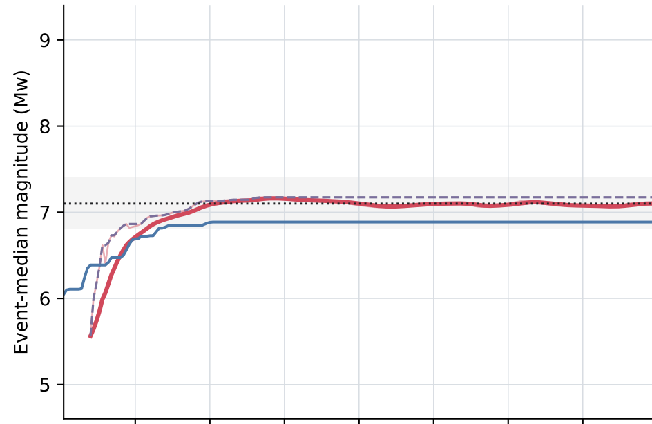
A. Anchorage2018 | Mw 7.10
