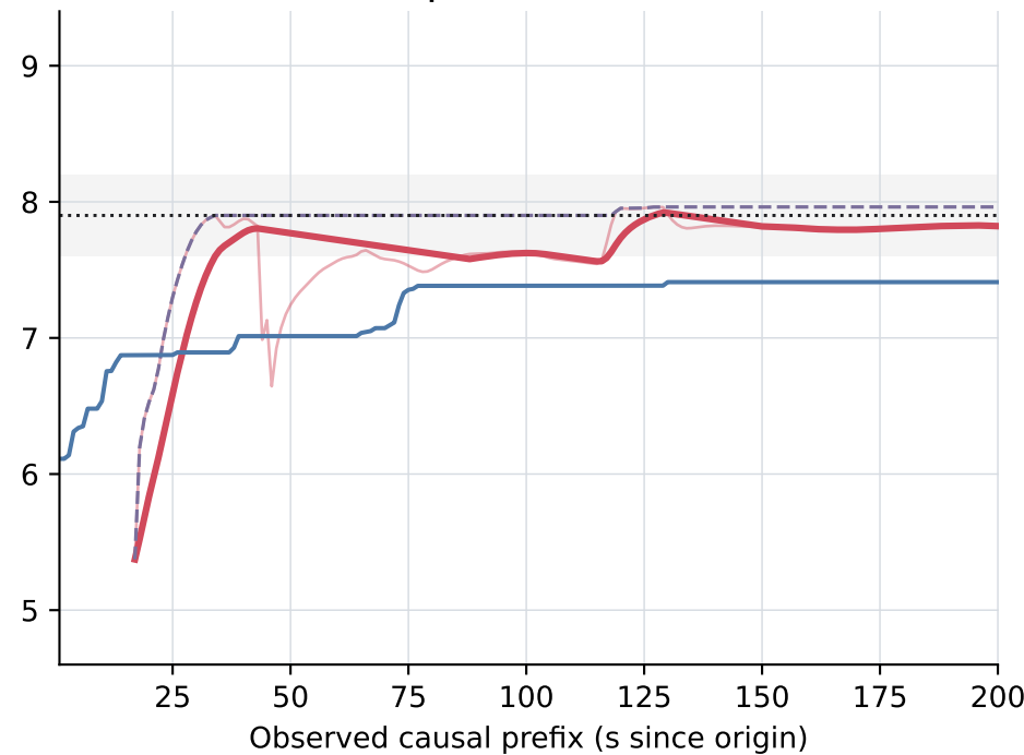
E. RatIslands2014 | Mw 7.90
