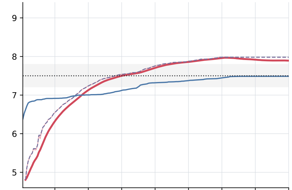
C. Noto2024 | Mw 7.50
