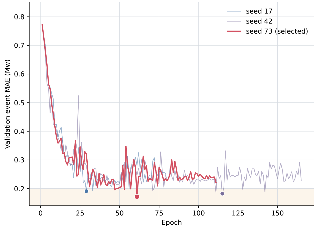
B. Validation trajectory
